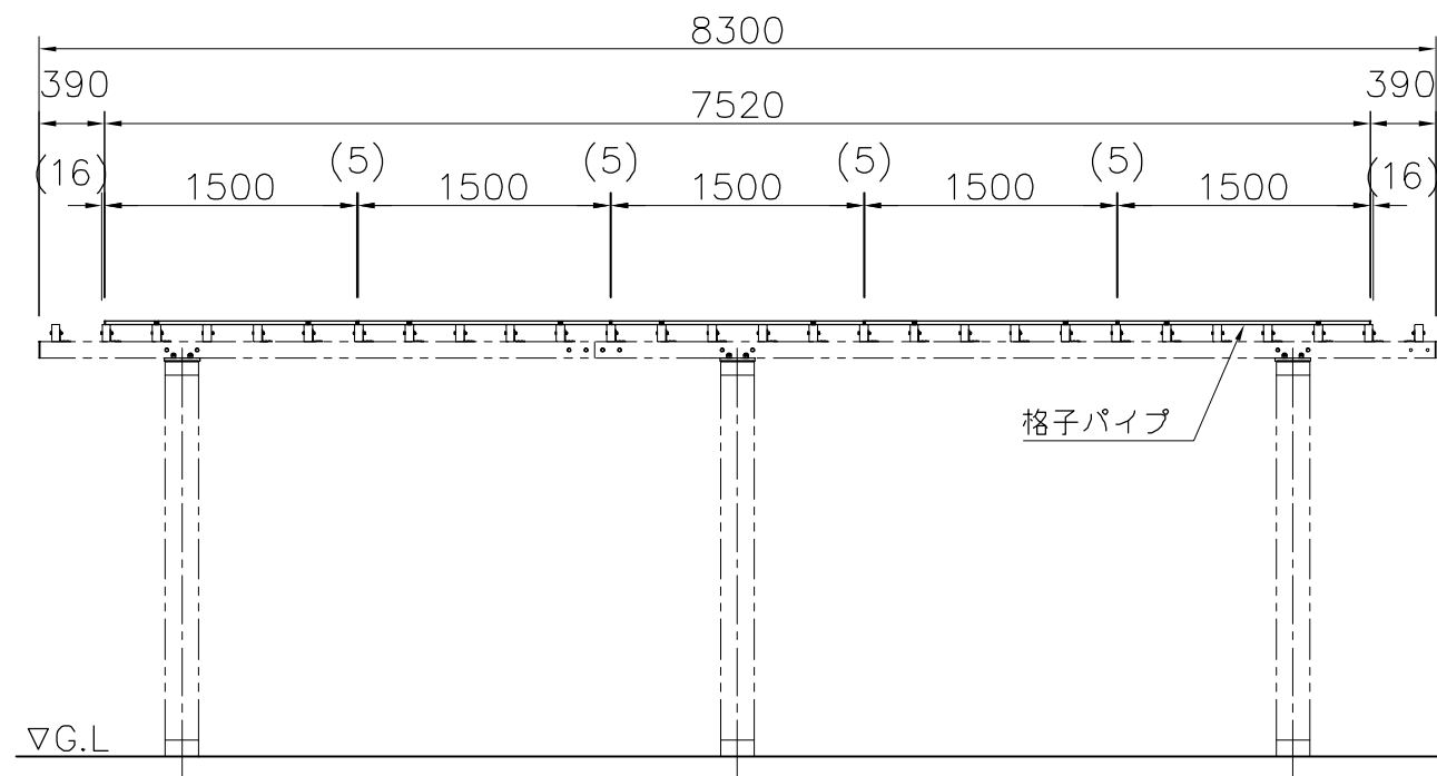
外観図 S=1/50
