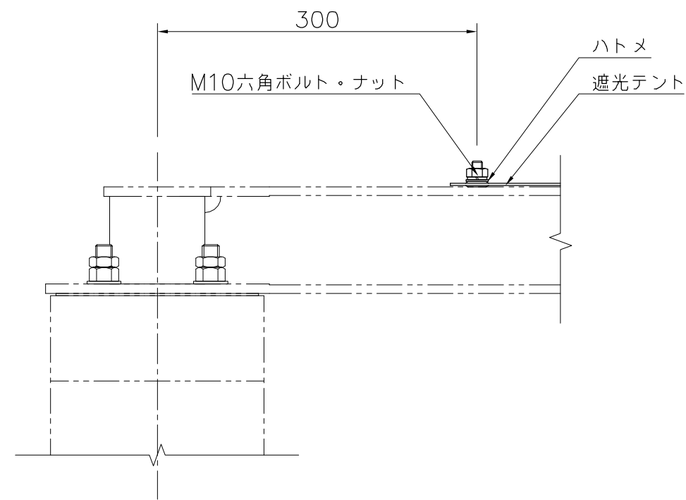
固定部詳細図 S=1/5
