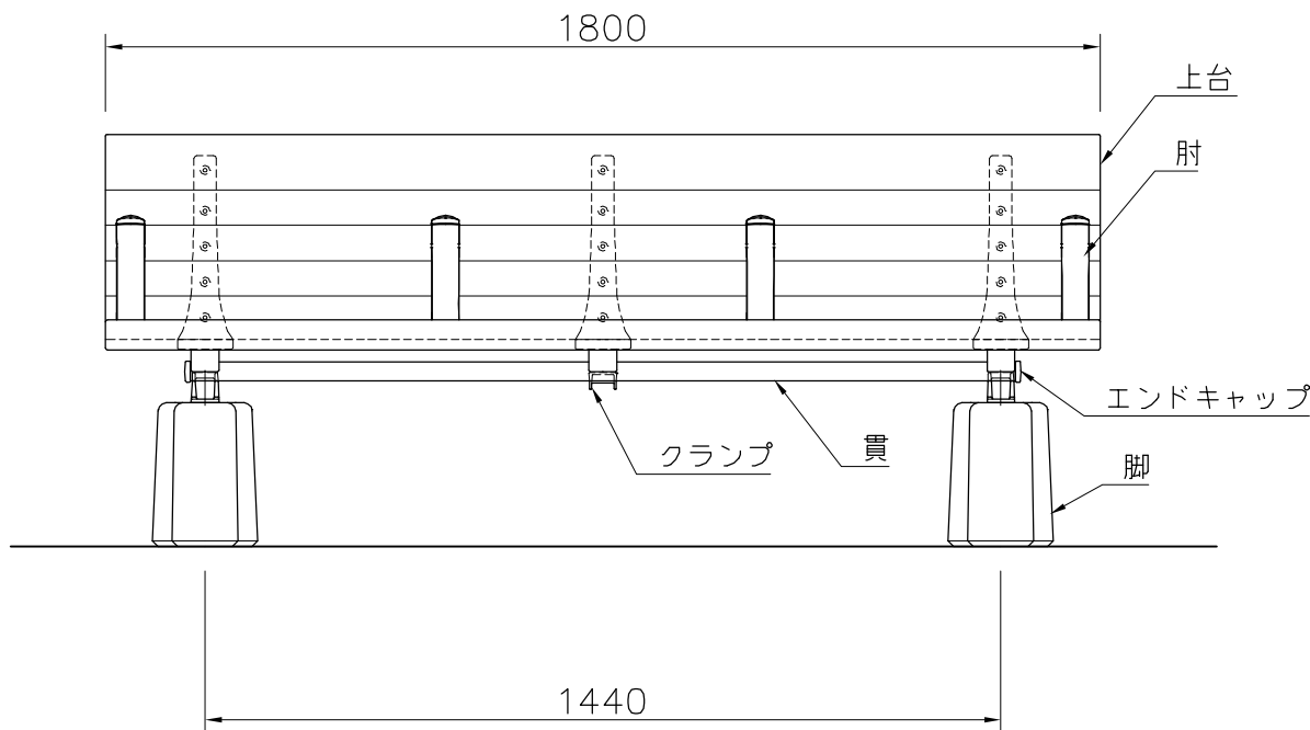
外観図 S=1/15
