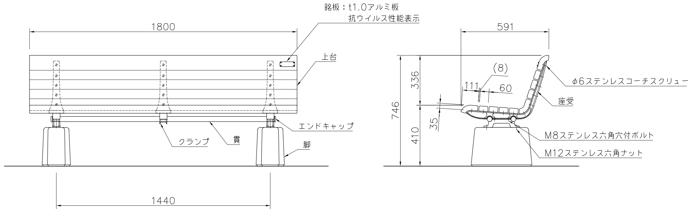
外観図 S=1/15
