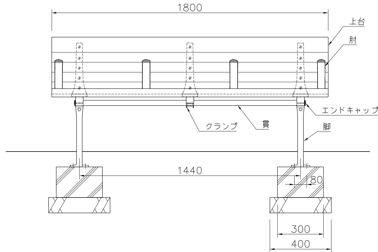
外観図 S=1/15
