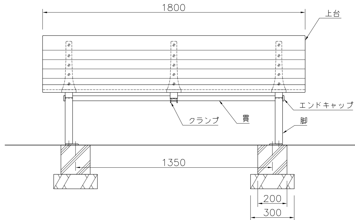
外観図 S=1/15
