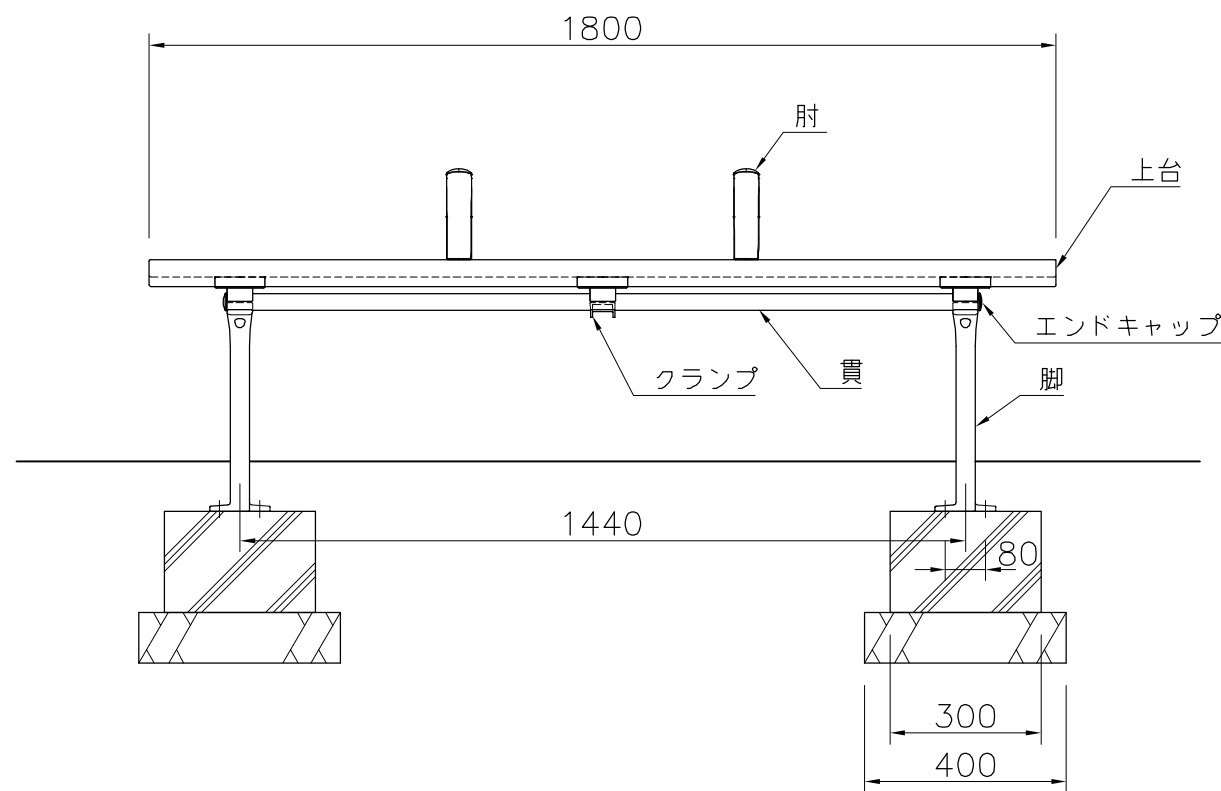
外観図 S=1/15
