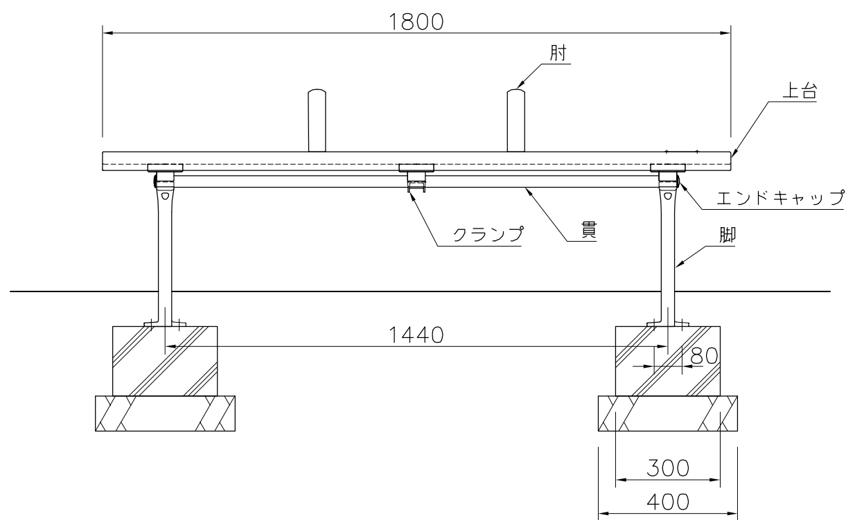
外観図 S=1/15
