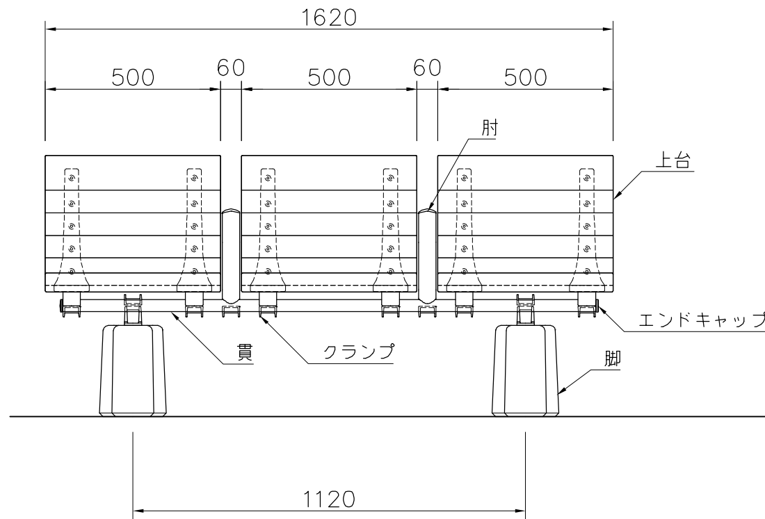
外観図 S=1/15
