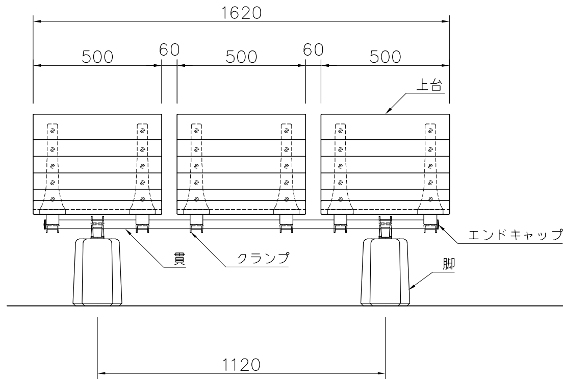
外観図 S=1/15
