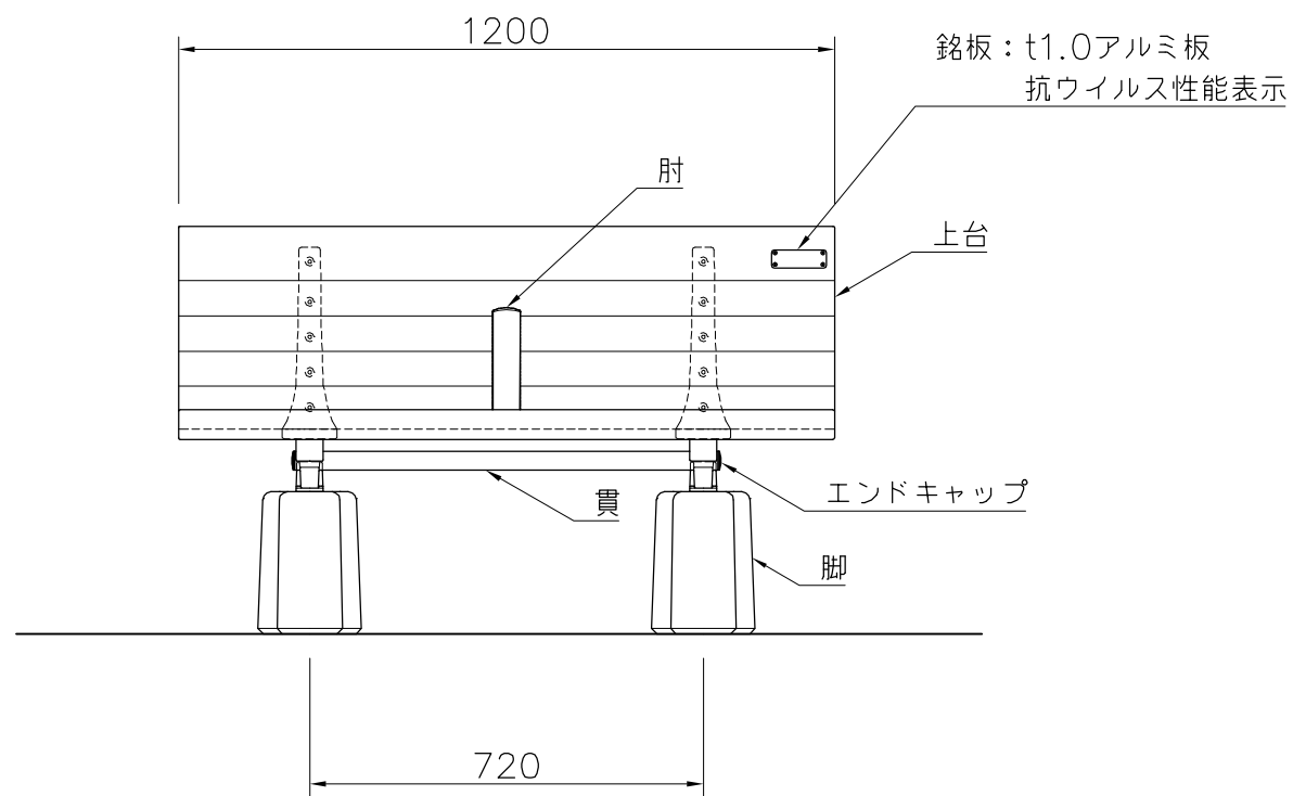
外観図 S=1/15
