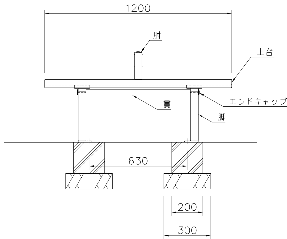
外観図 S=1/15
