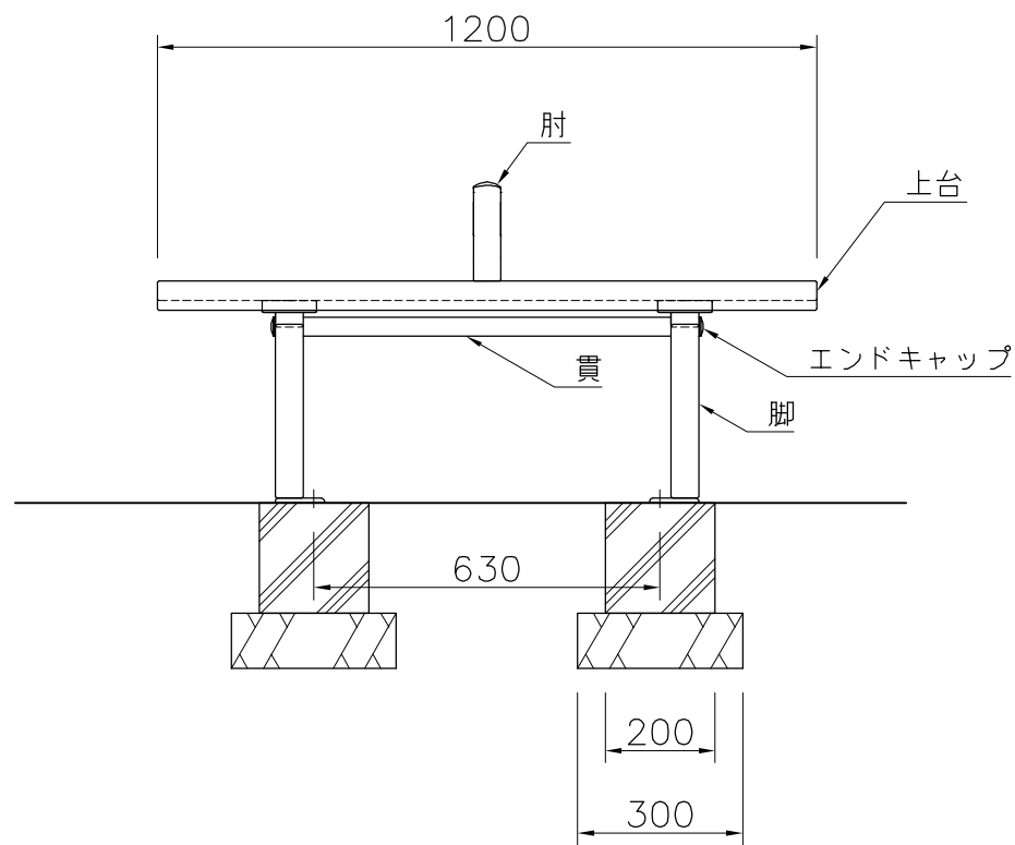
外観図 S=1/15
