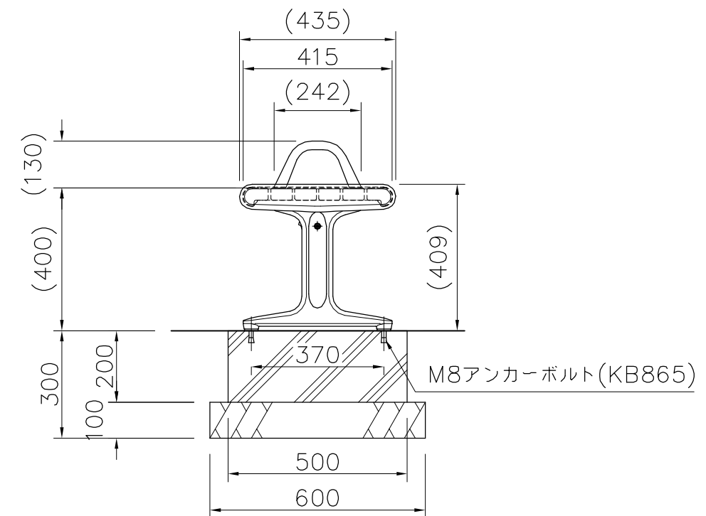
外観図 S=1/15
