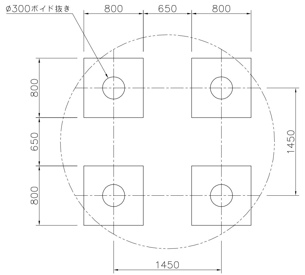
基礎伏図 S=1/30
