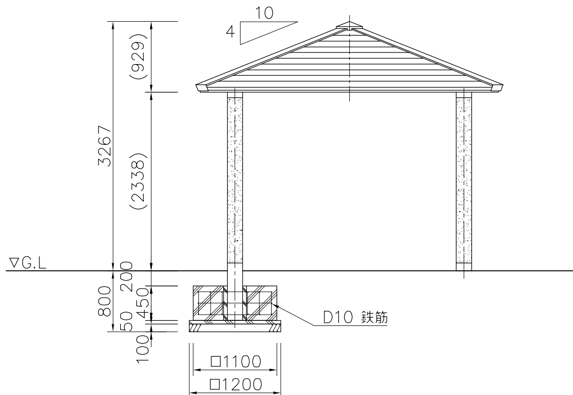
外観図 S=1/50
