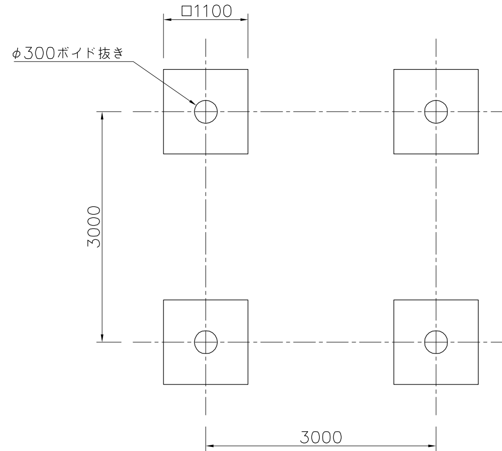
基礎伏図 S=1/50
