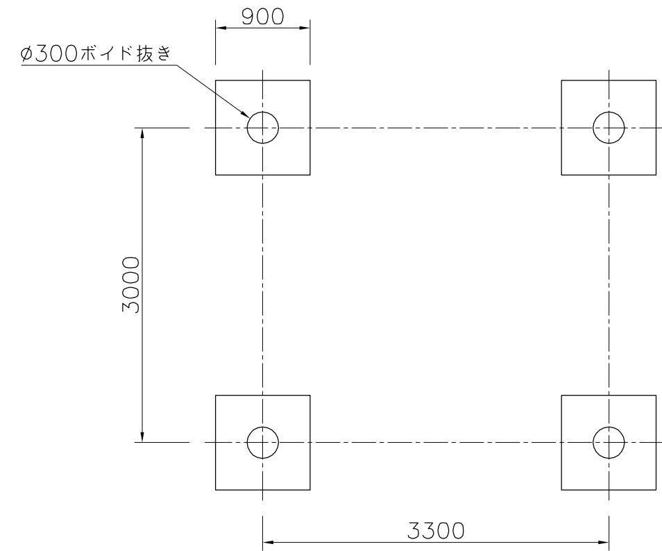
基礎伏図 1/50
