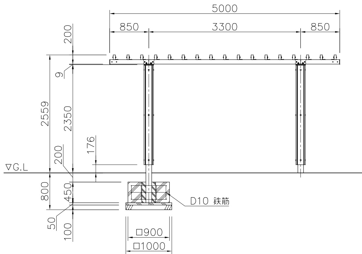
外観図 1/50
