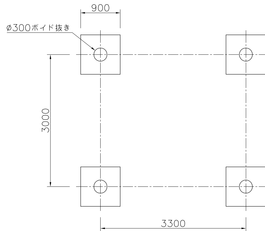
基礎伏図 1/50
