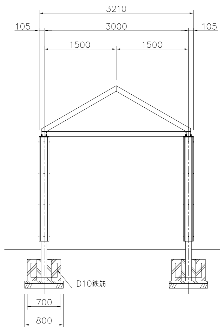
外観図 S=1/40
