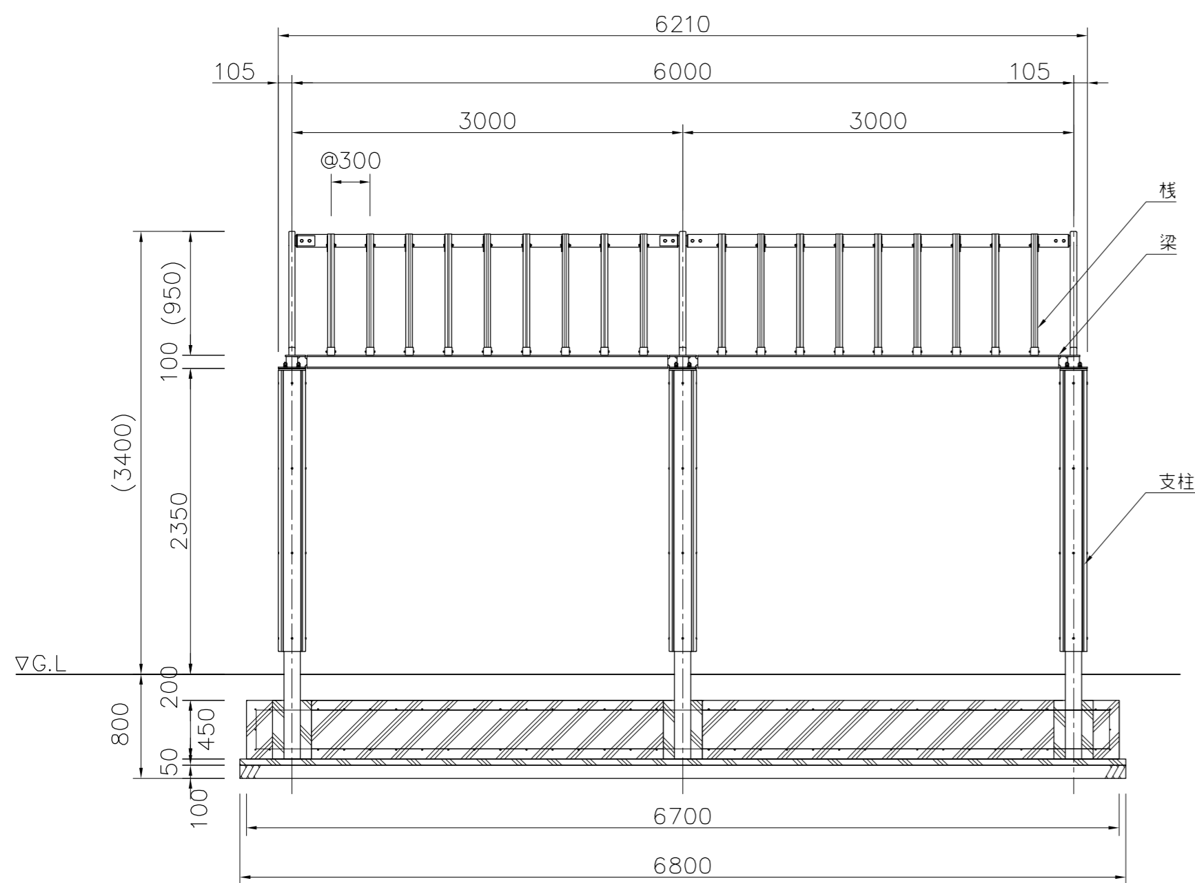
外観図 S=1/40
