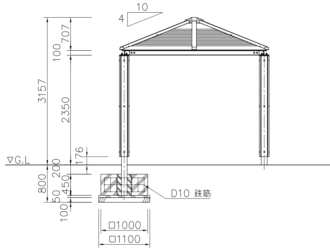
外観図 S=1/50
