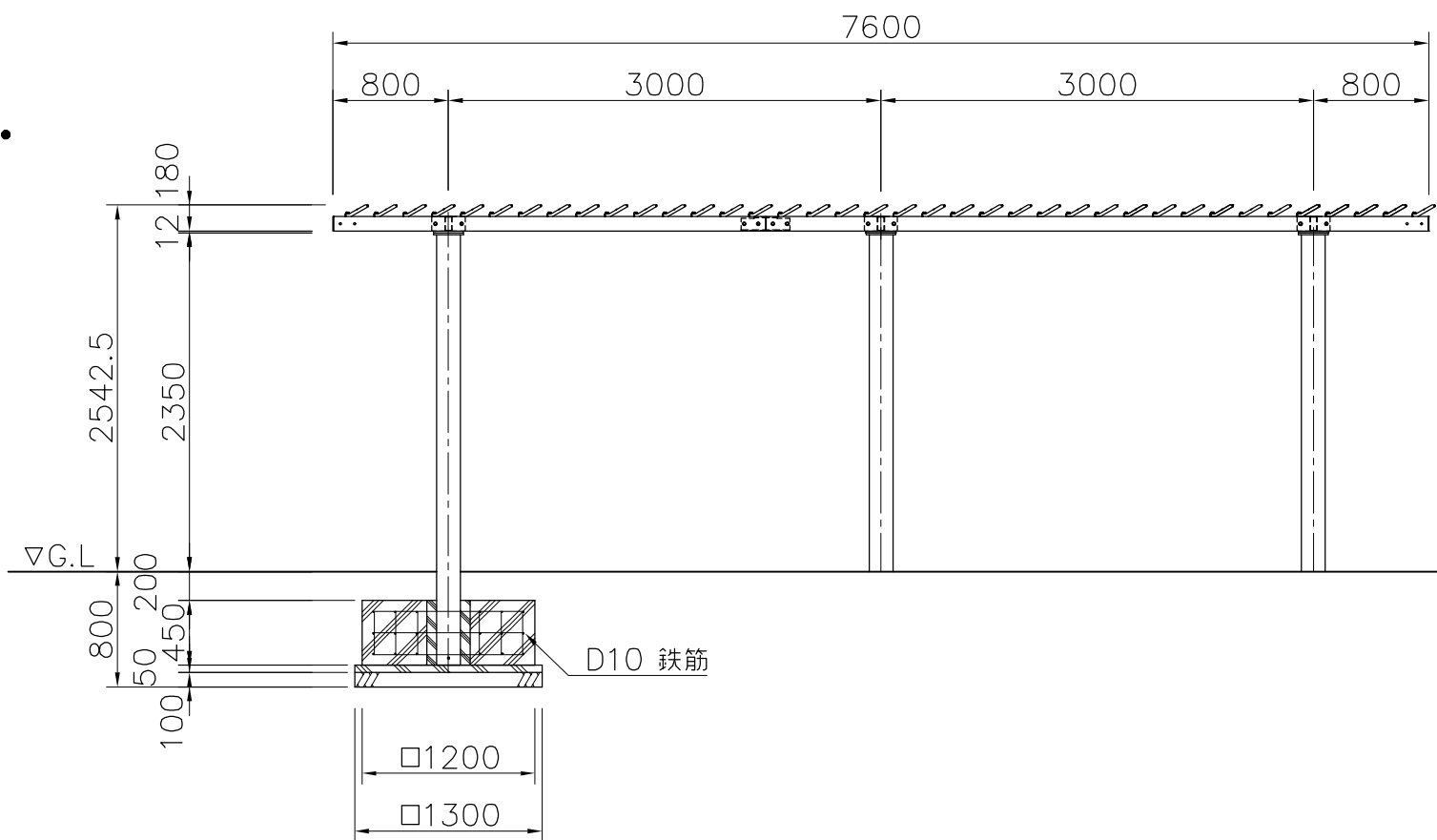
外観図 S=1/50
