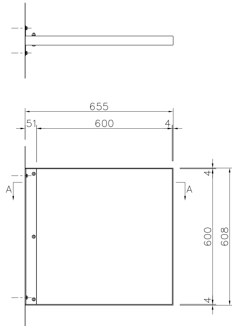
外観図 S=1/10
