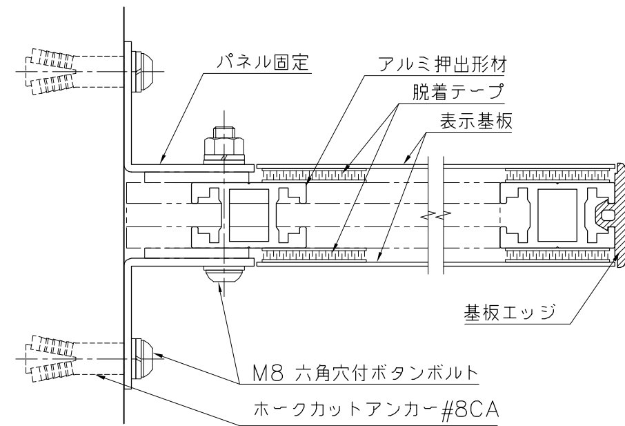
A-A断面図 S=1/2
