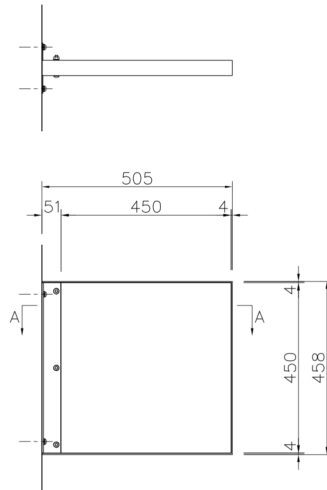
外観図 S=1/10
