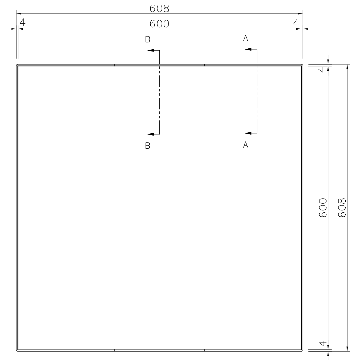
外観図 S=1/5
