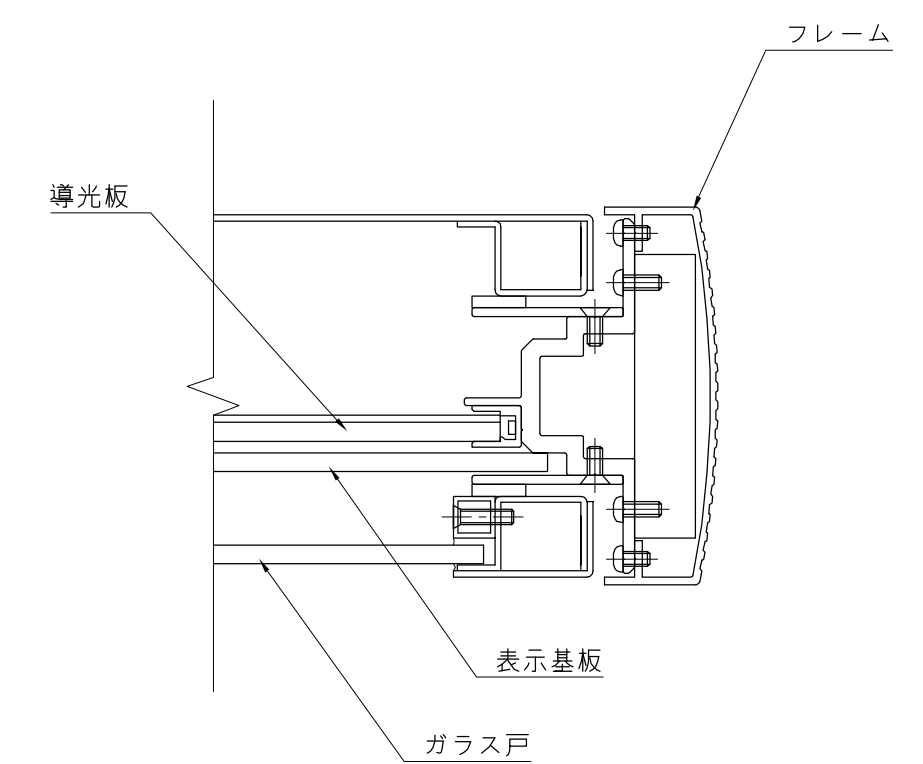
A断面詳細図 S=1/2
