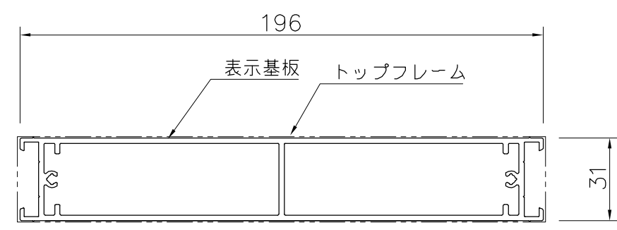
A断面図 S=1/2
