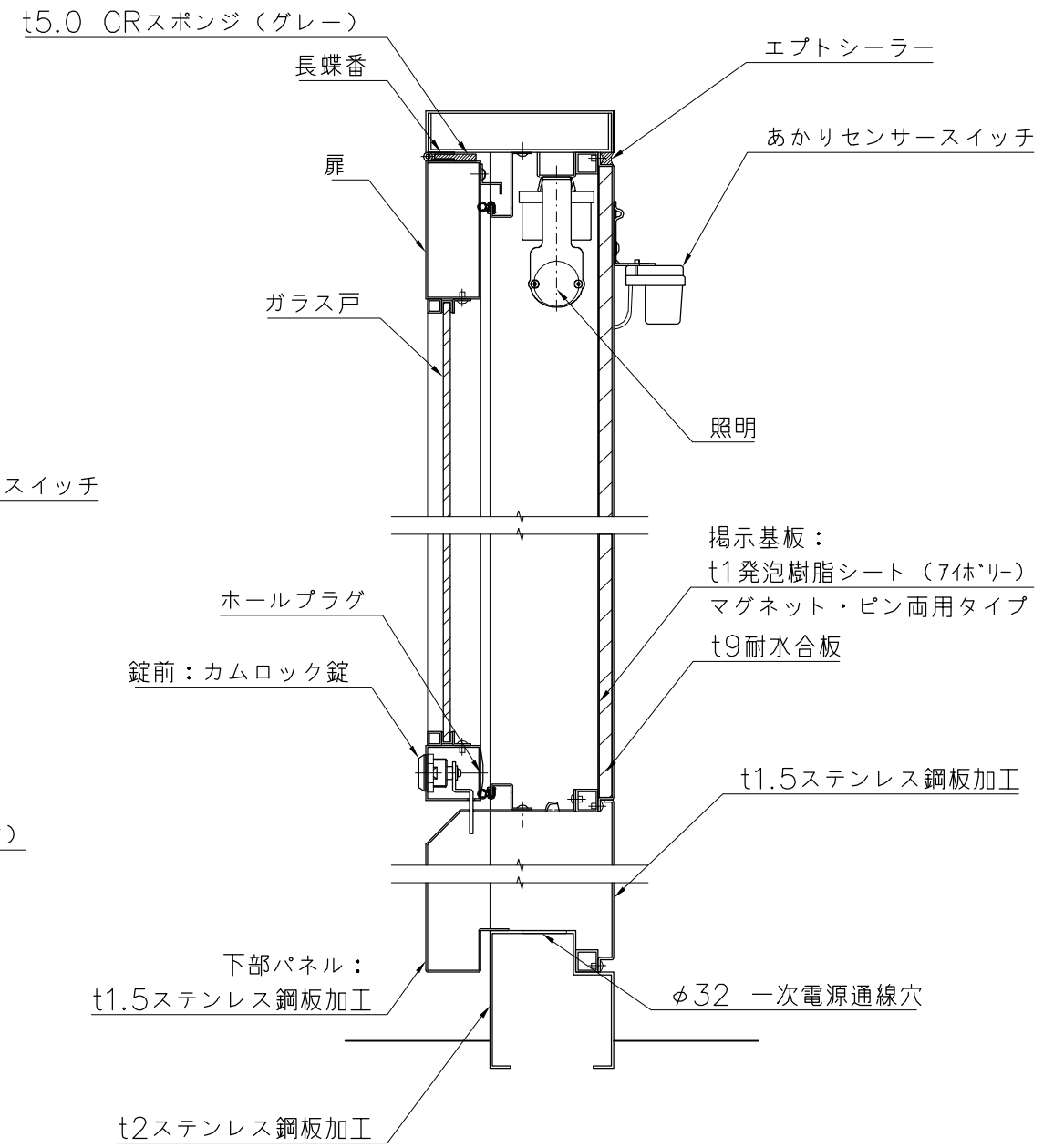
A断面詳細図 S=1/5
