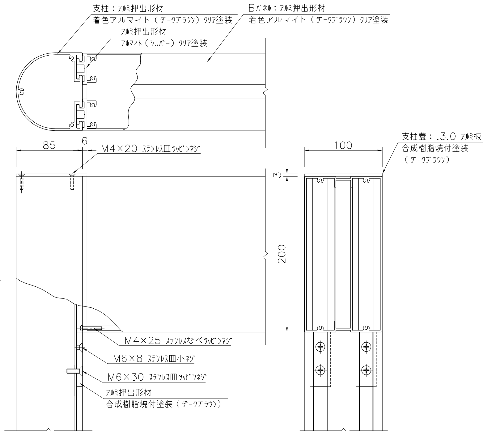
詳細図 S=1/3
