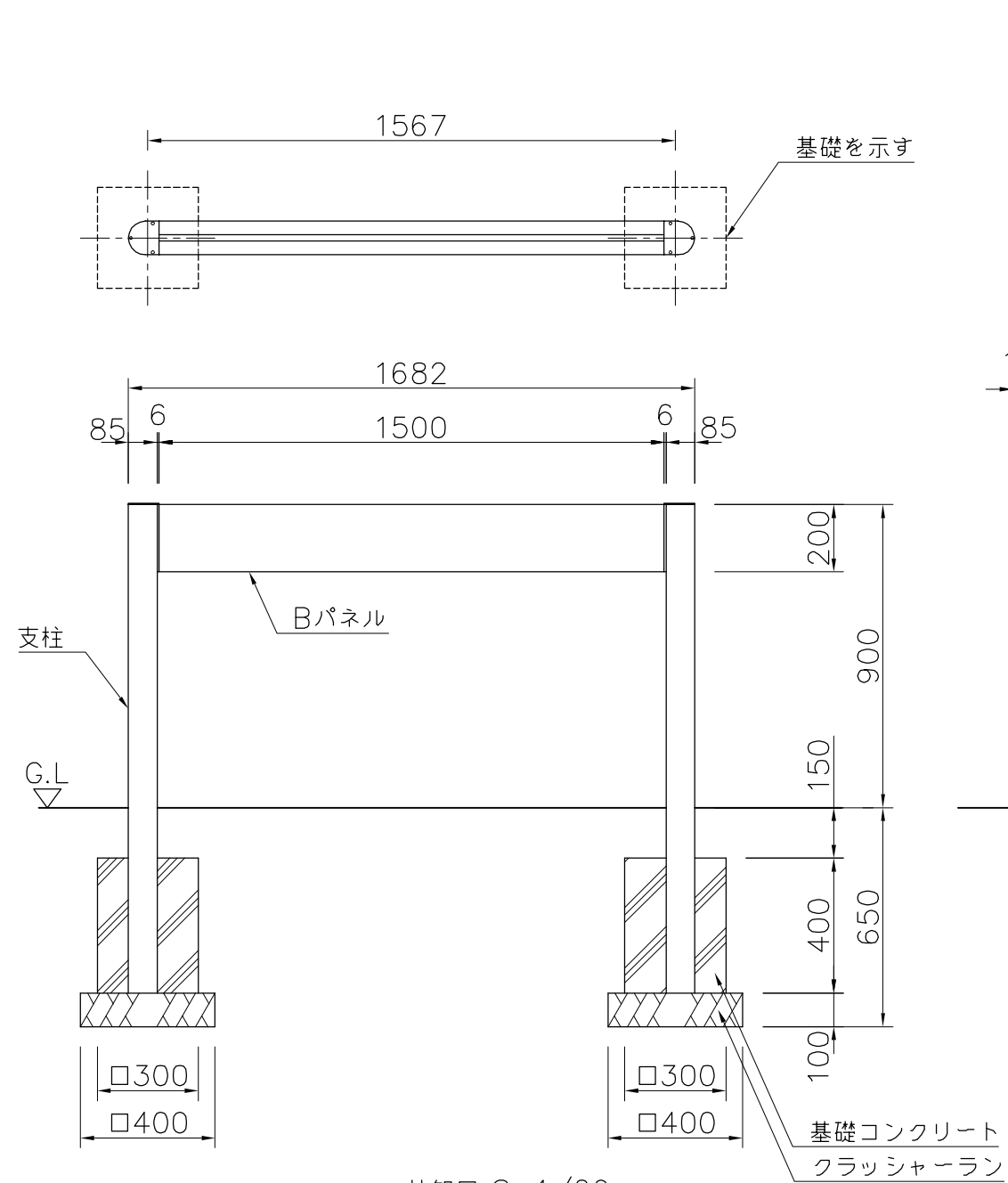
外観図 S=1/20
