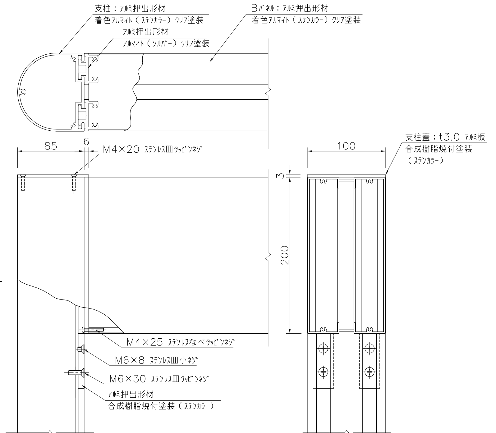
詳細図 S=1/3
