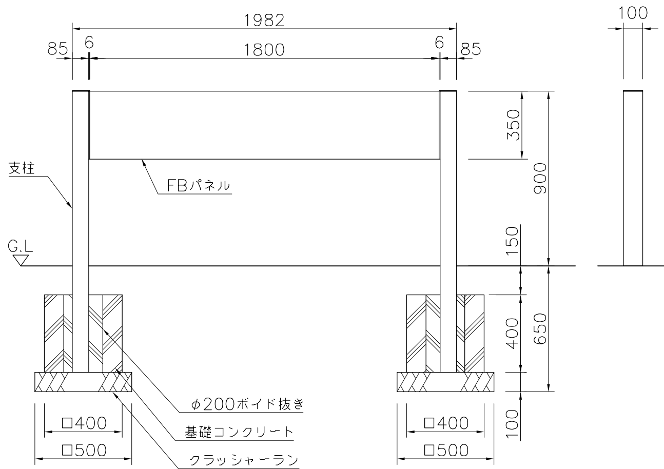
外観図 S=1/20
