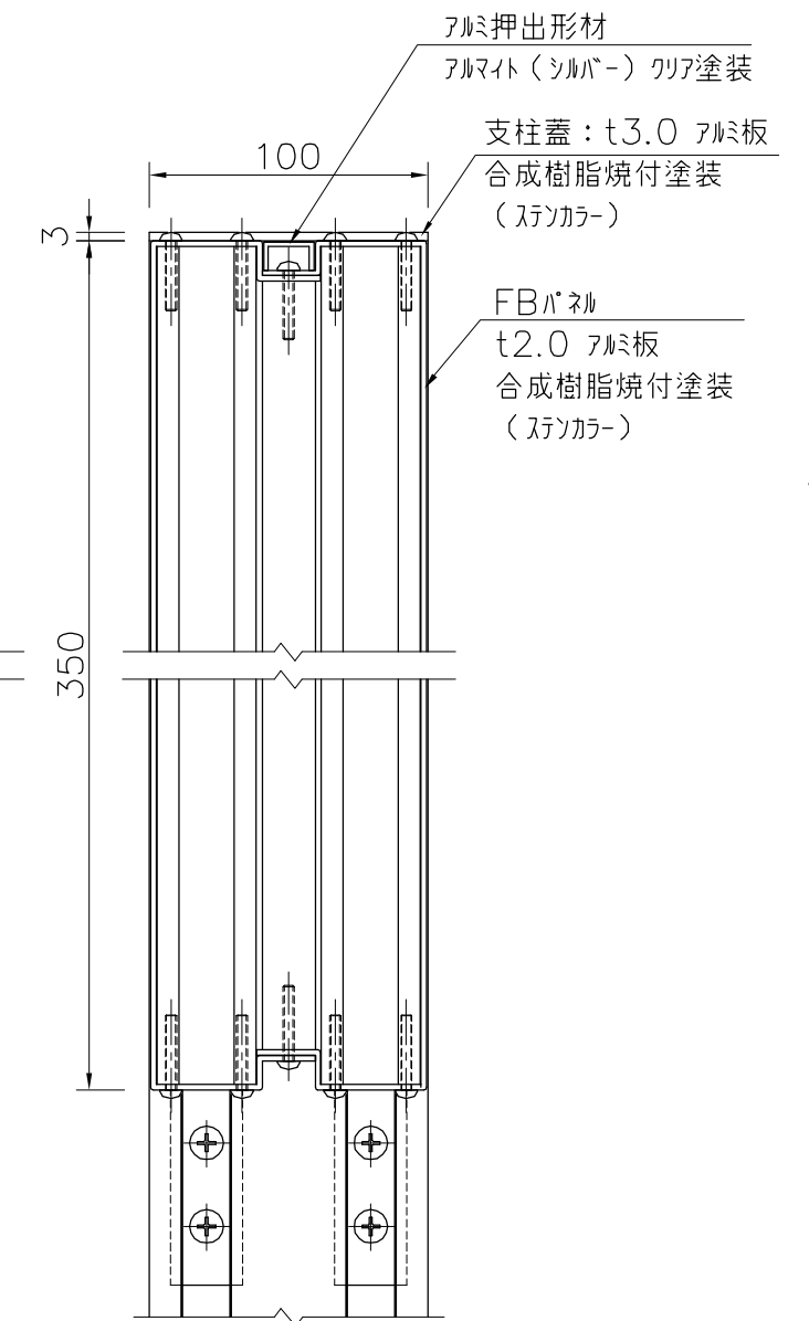
詳細図 S=1/3
