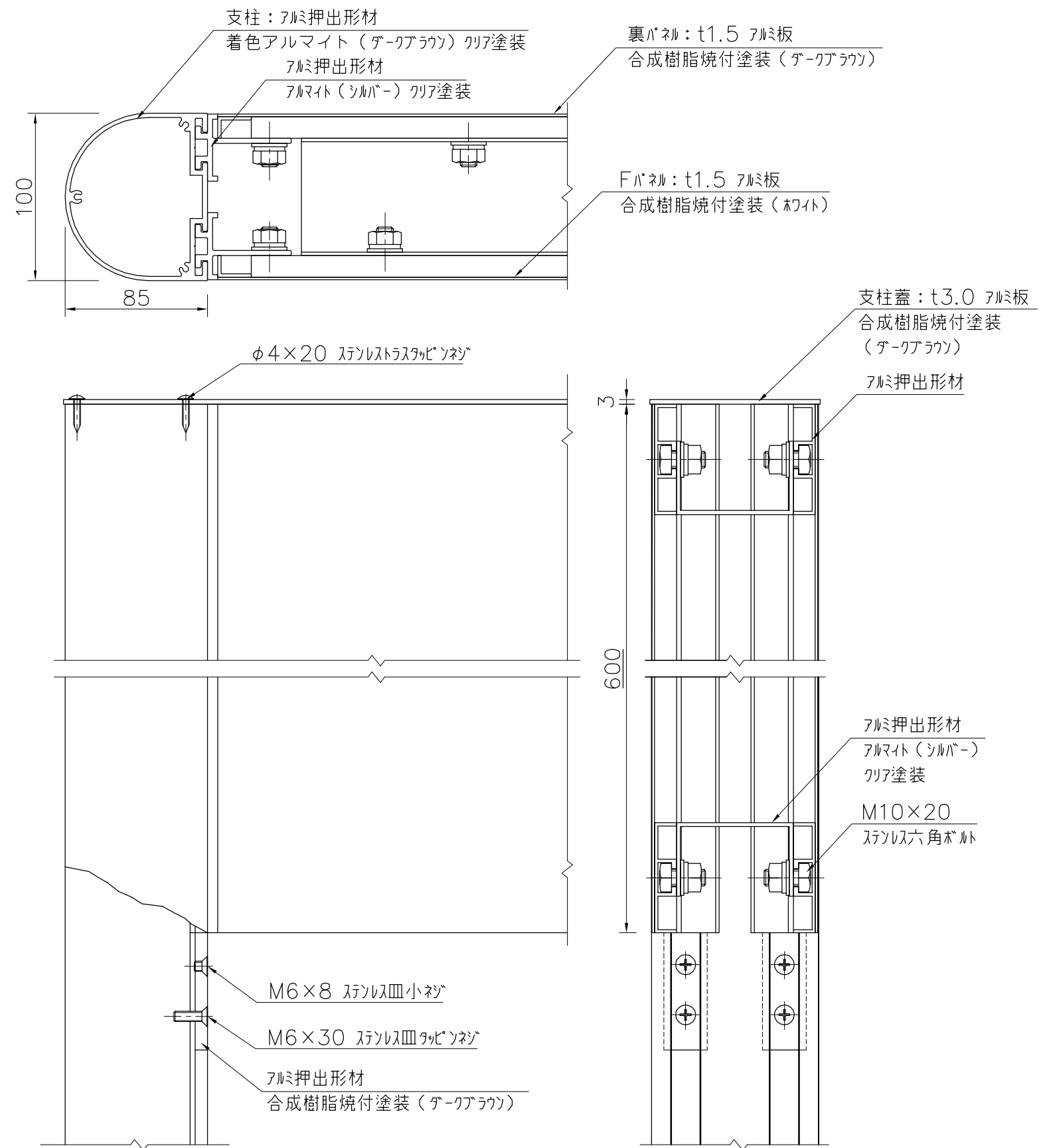
詳細図 S=1/3
