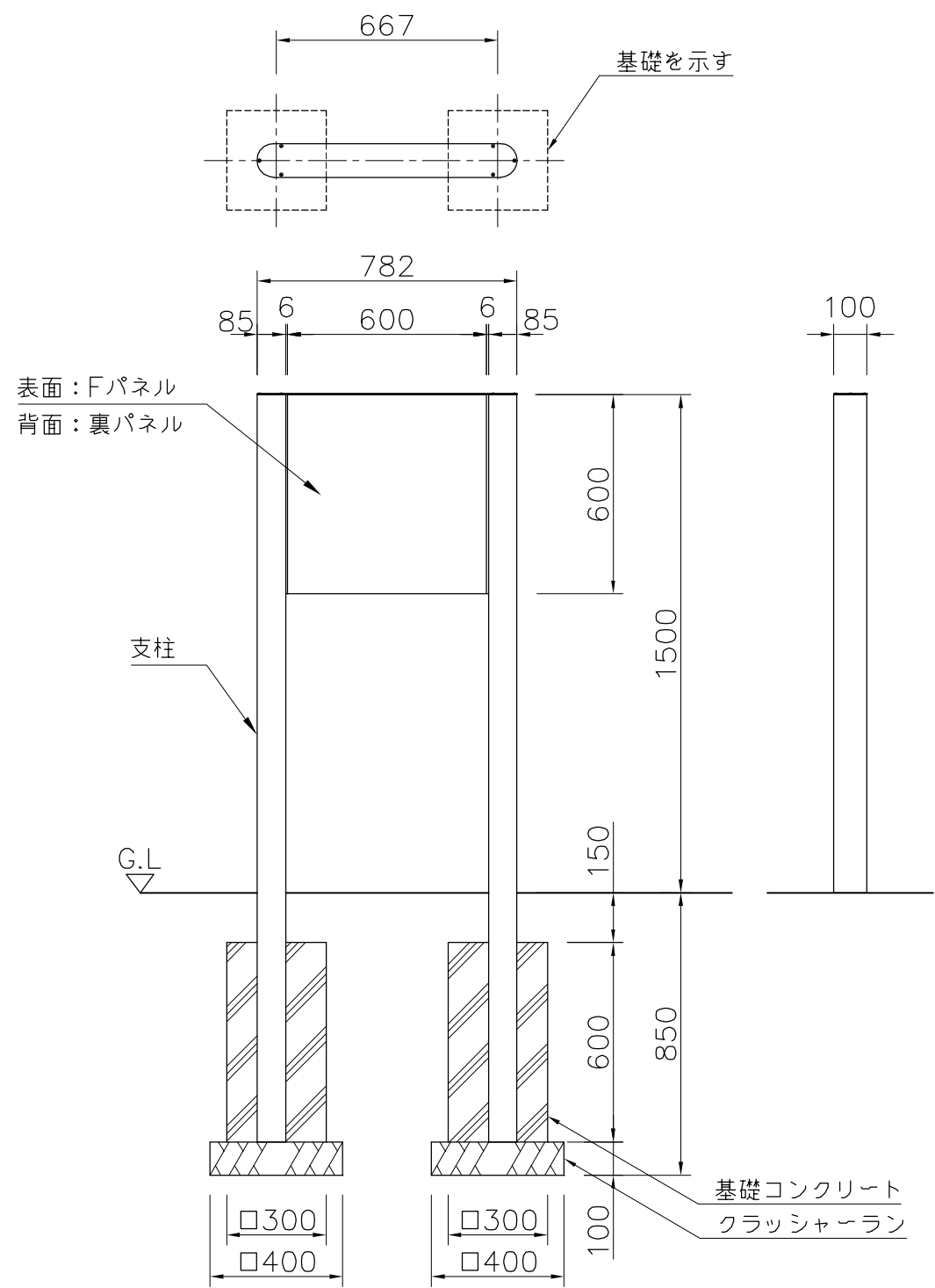
外観図 S=1/20
