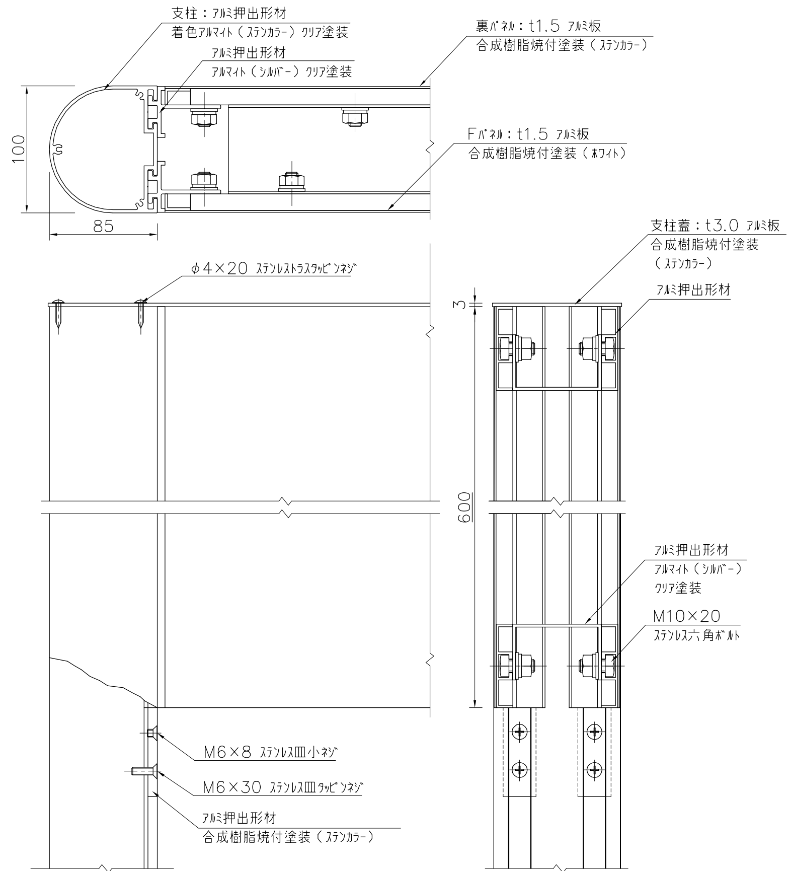
詳細図 S=1/3
