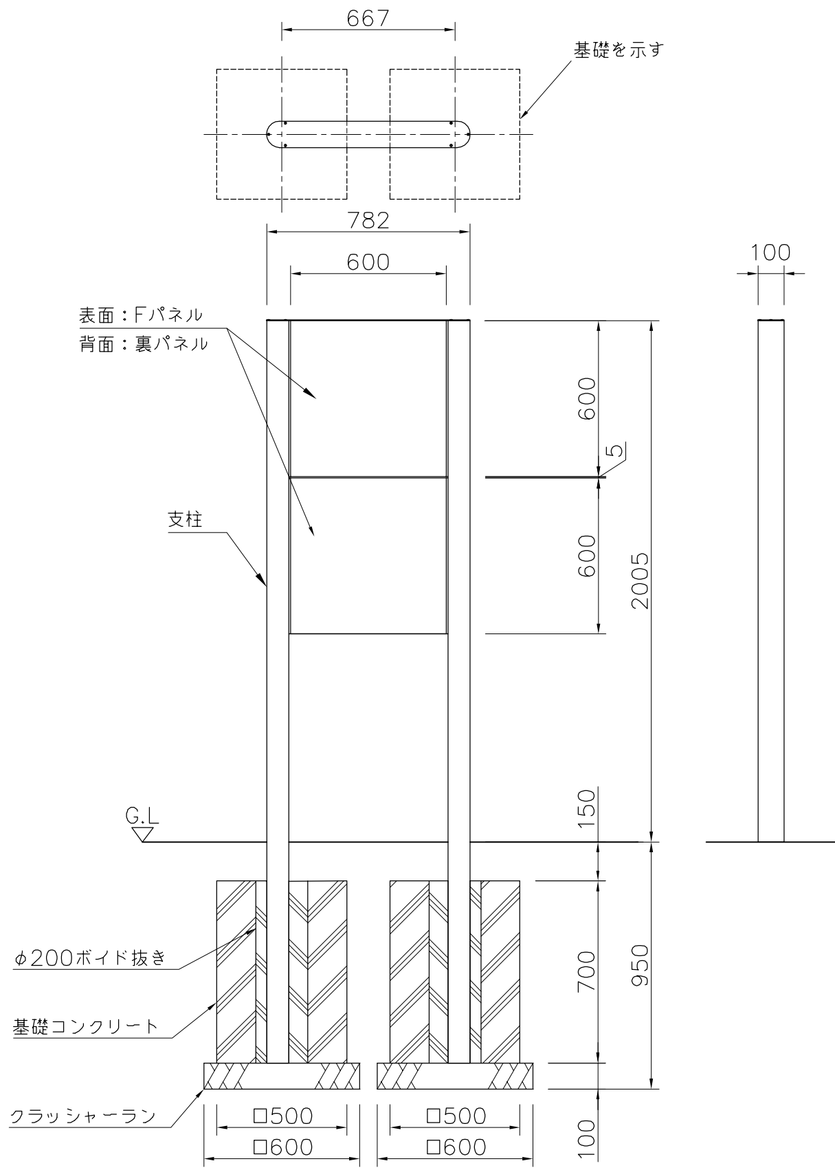
外観図 S=1/20
