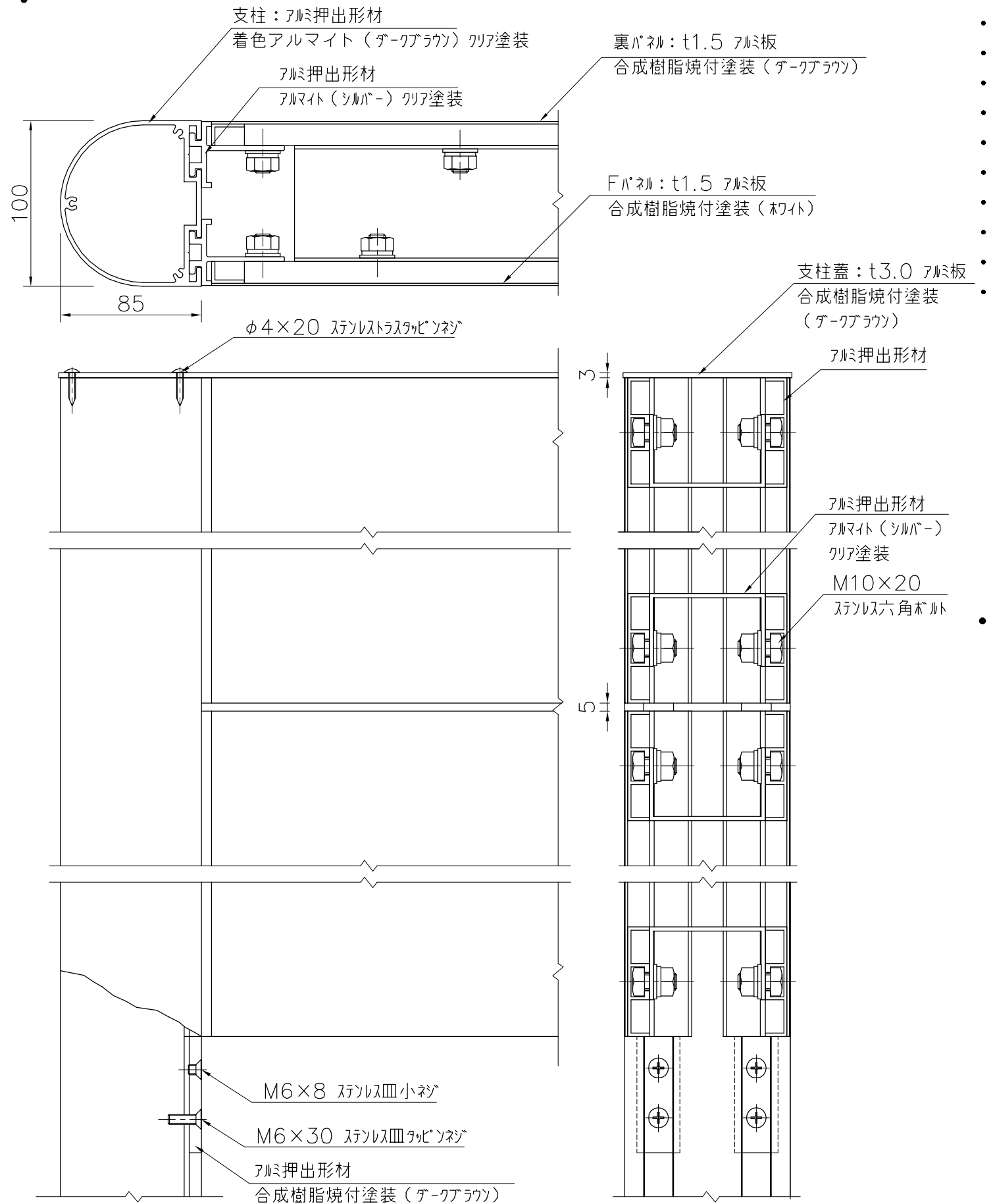
詳細図 S=1/3
