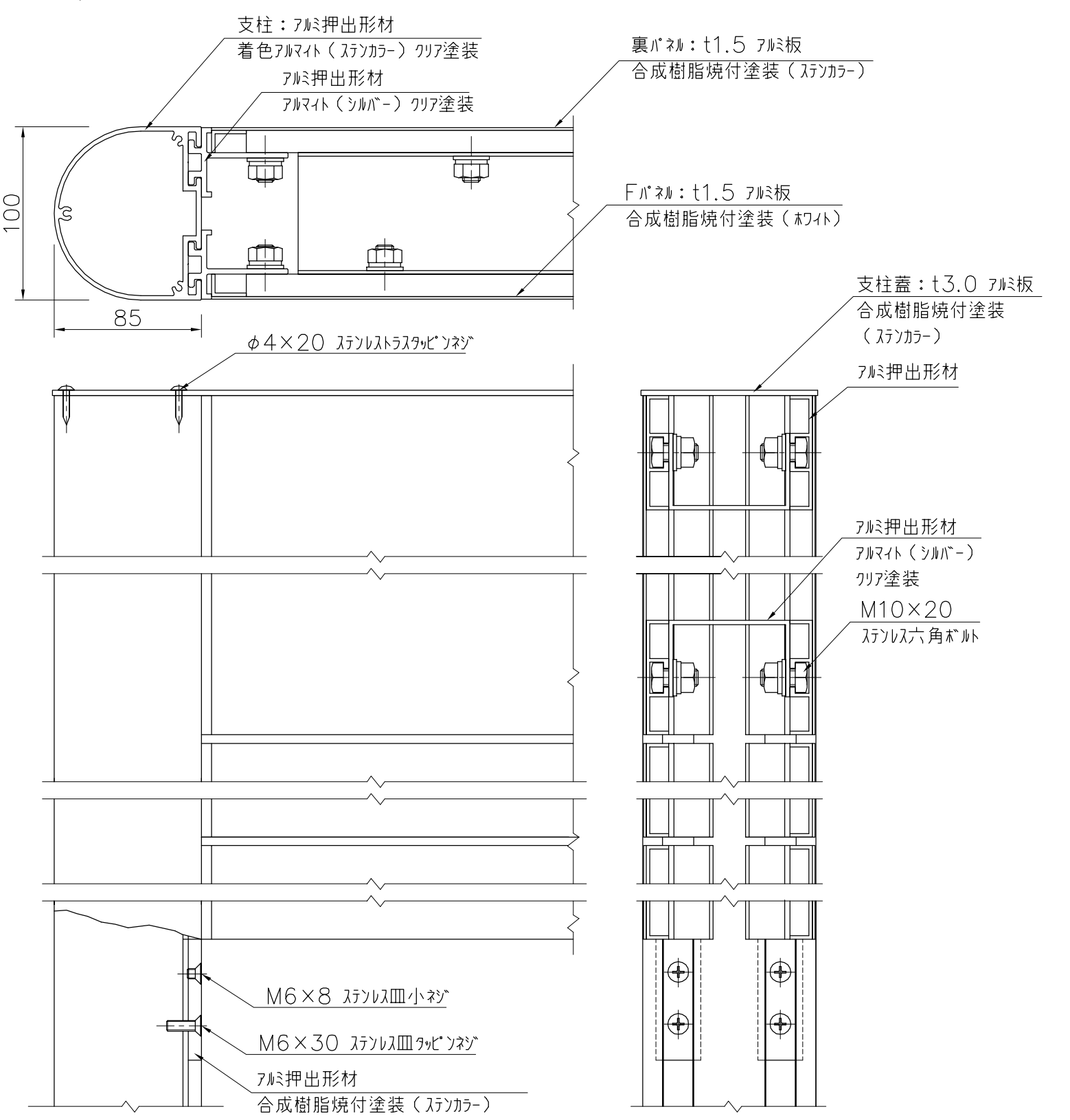
詳細図 S=1/3
