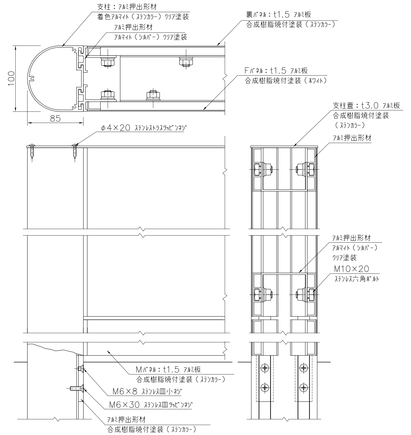
詳細図 S=1/3
