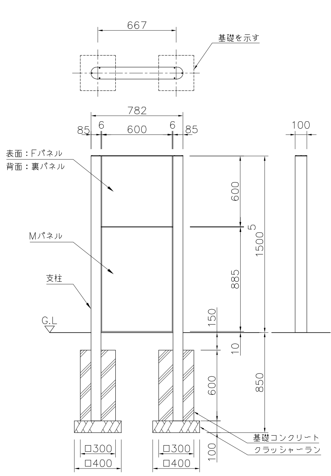
外観図 S=1/20
