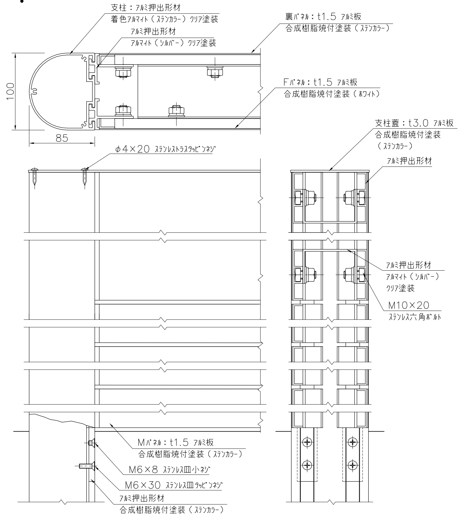
詳細図 S=1/3
