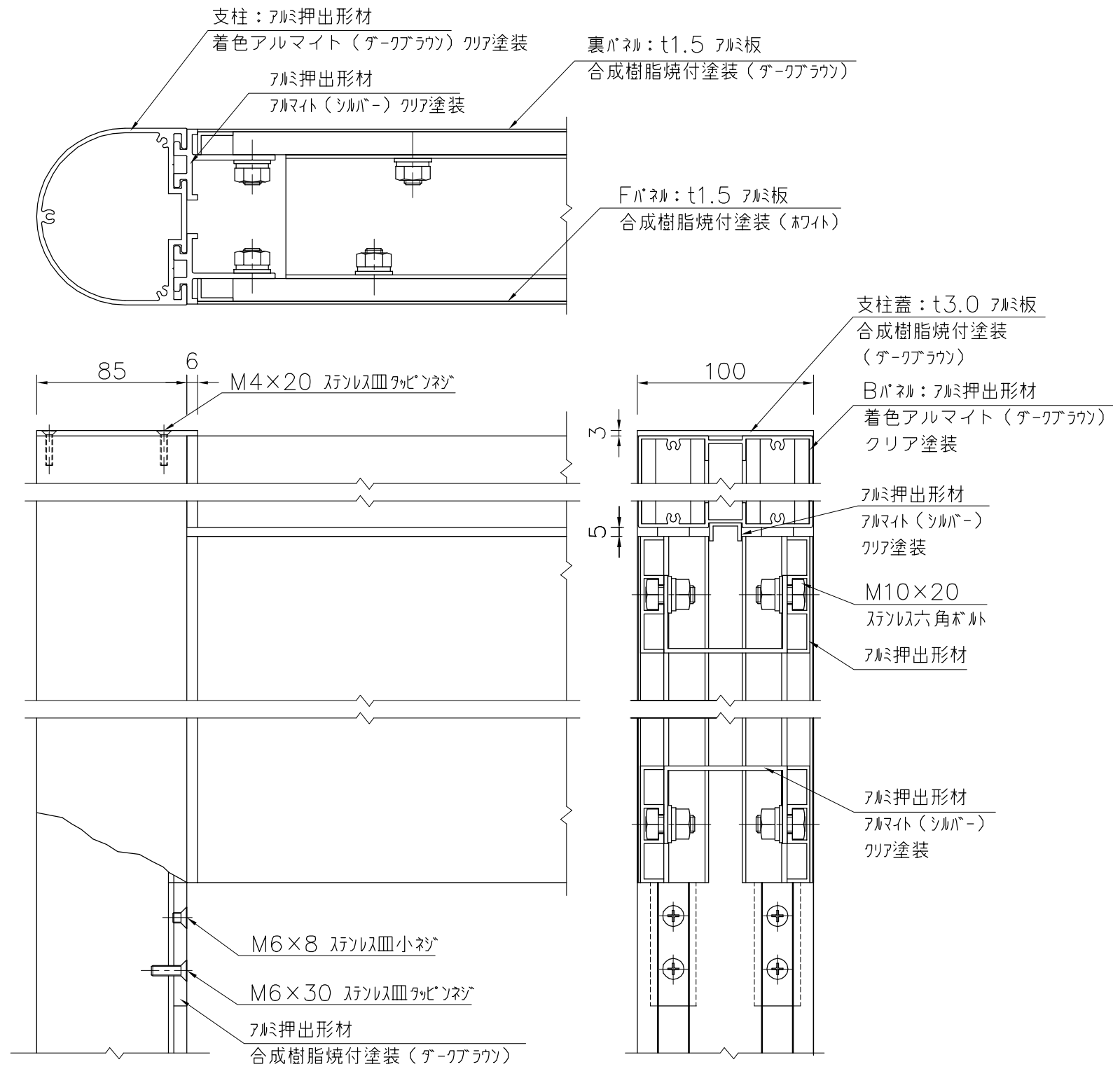
詳細図 S=1/3
