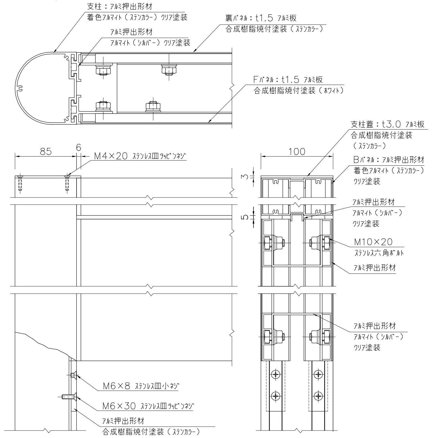
詳細図 S=1/3
