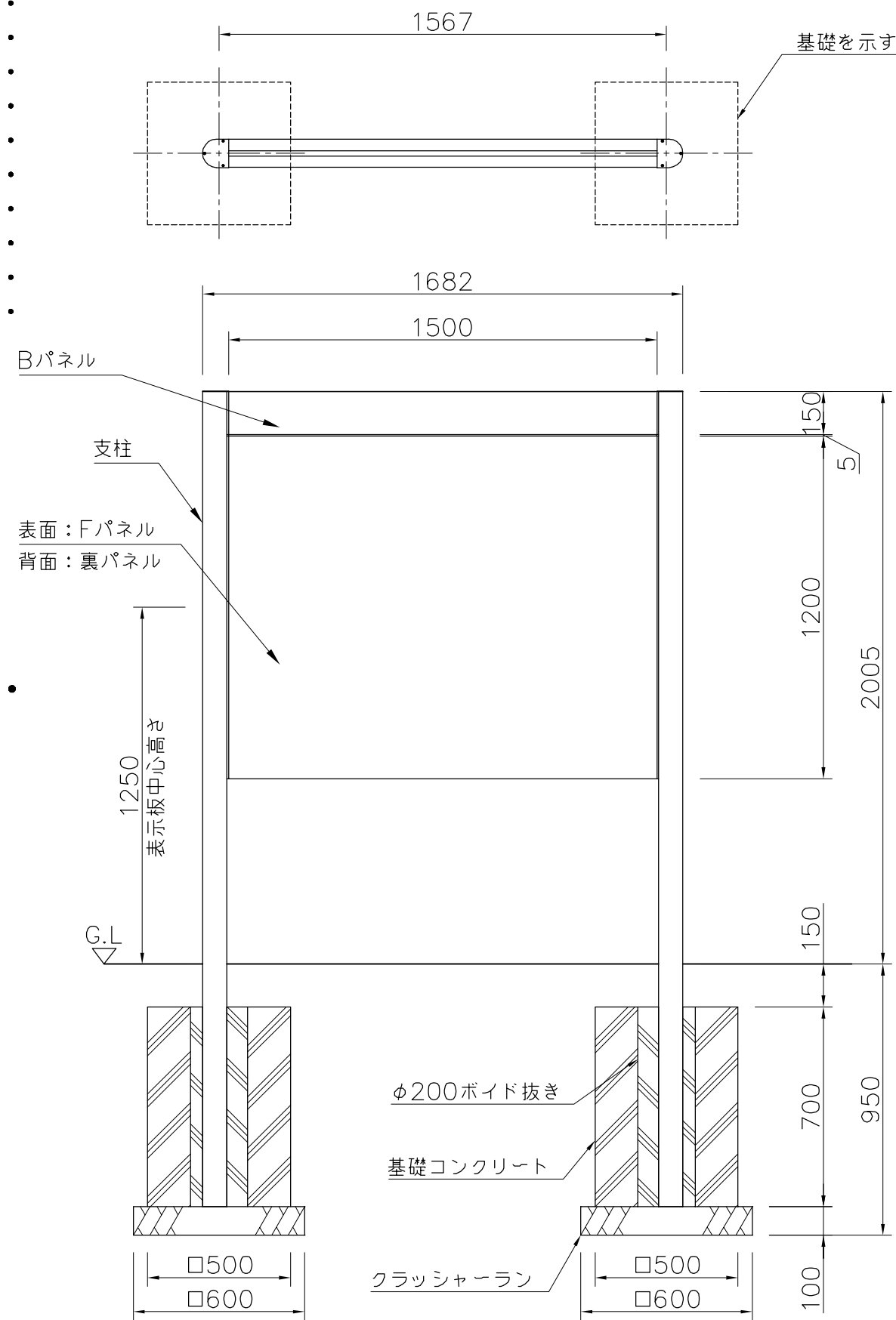
外観図 S=1/20
