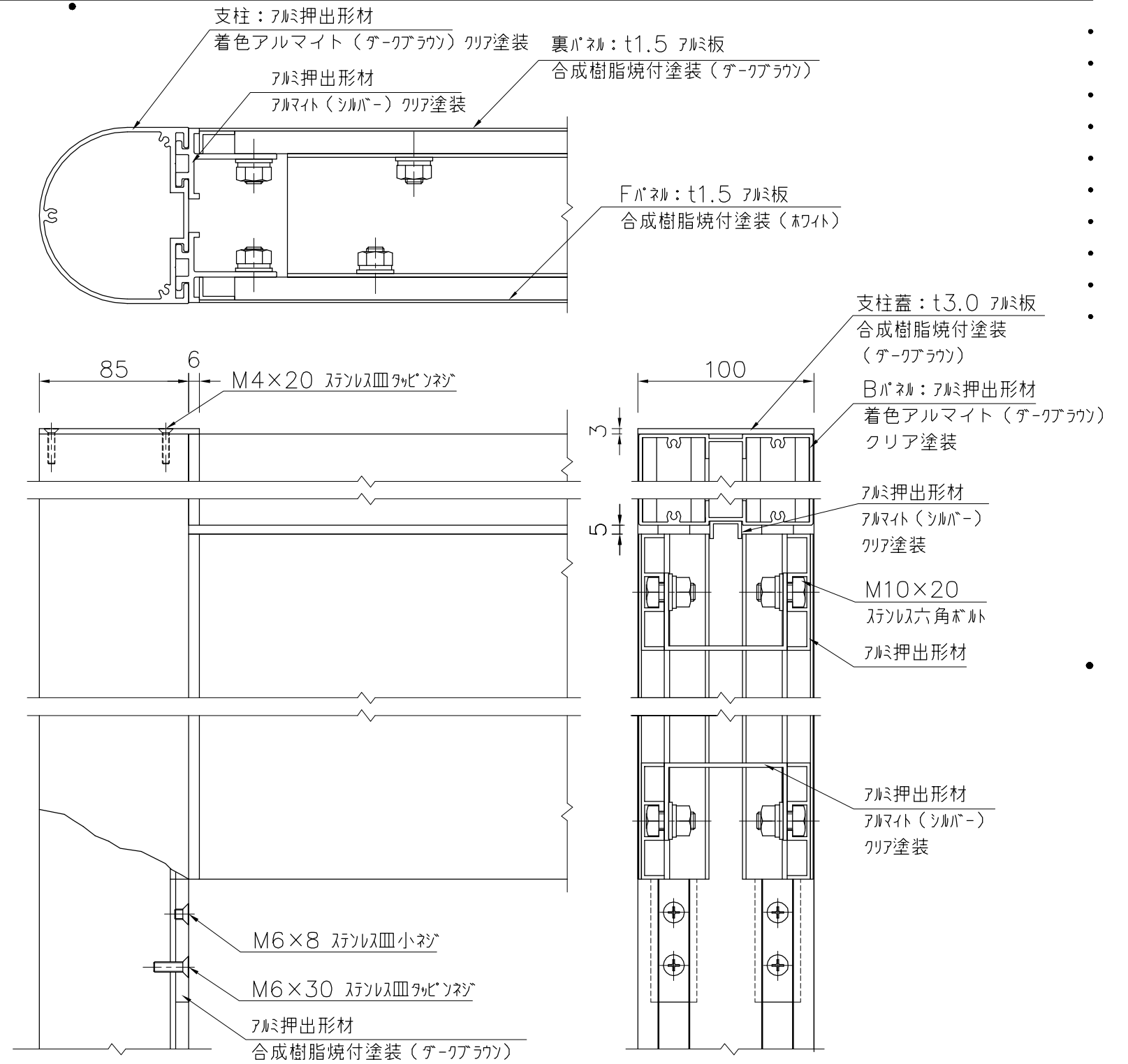
詳細図 S=1/3
