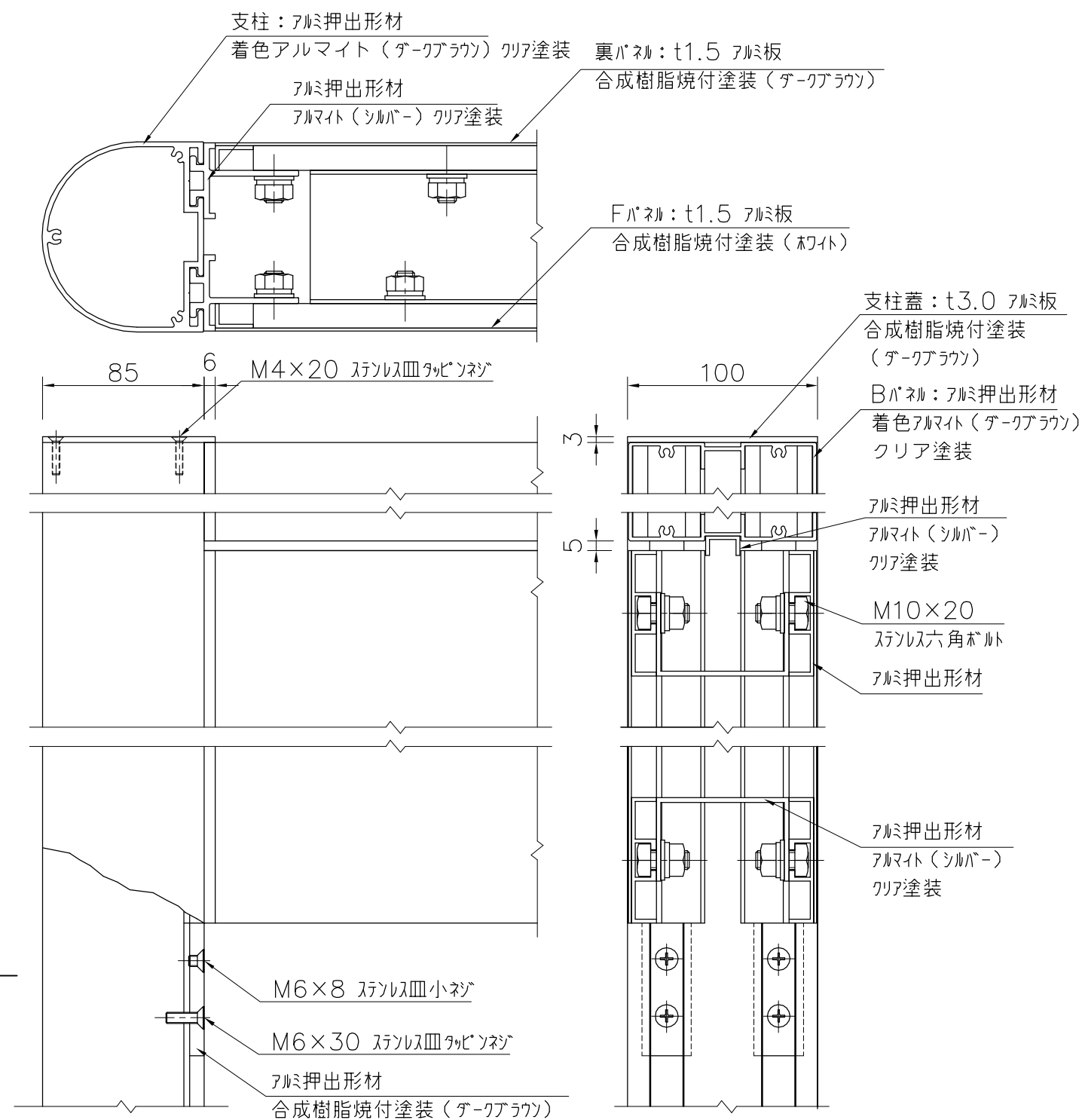
詳細図 S=1/3
