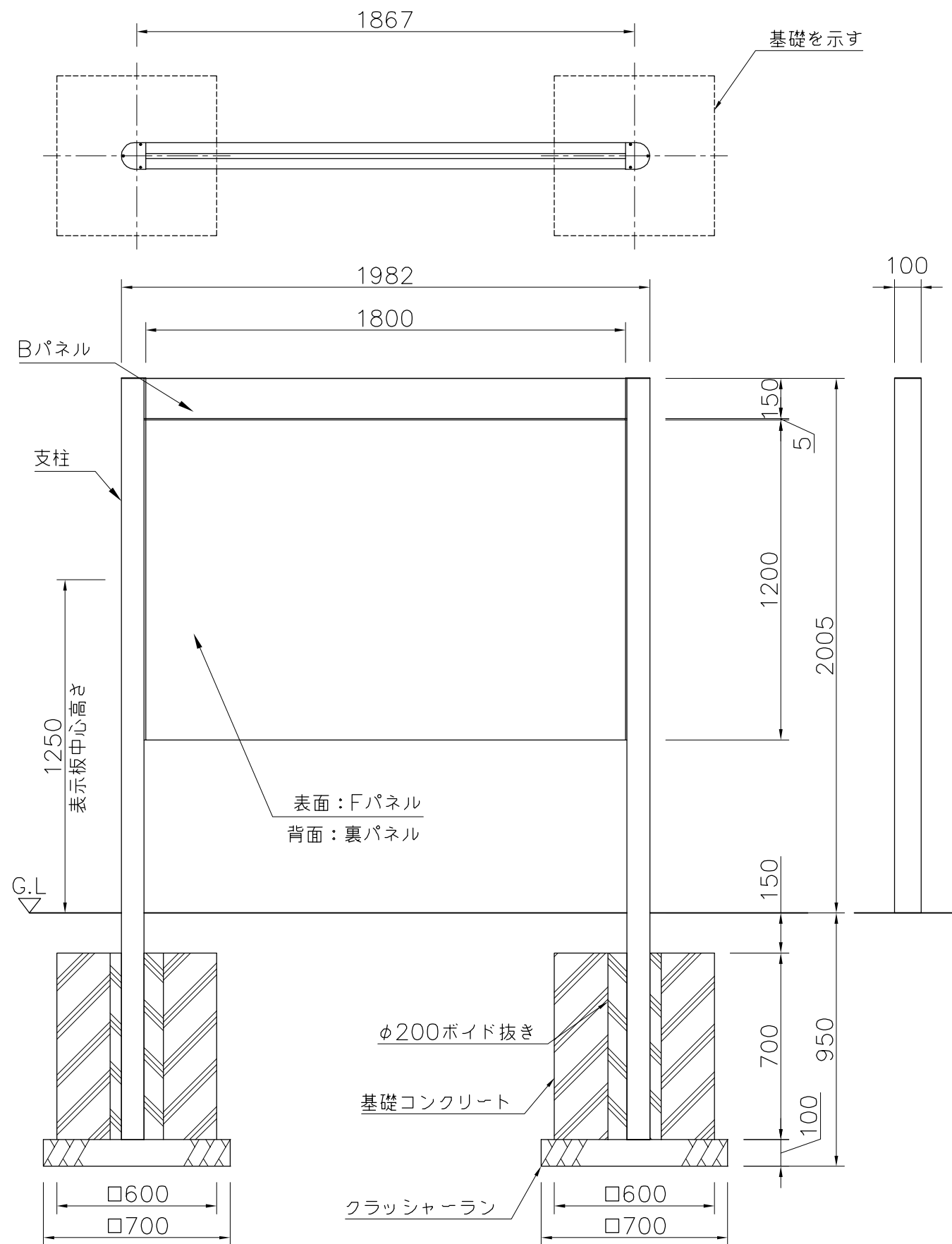
外観図 S=1/20
