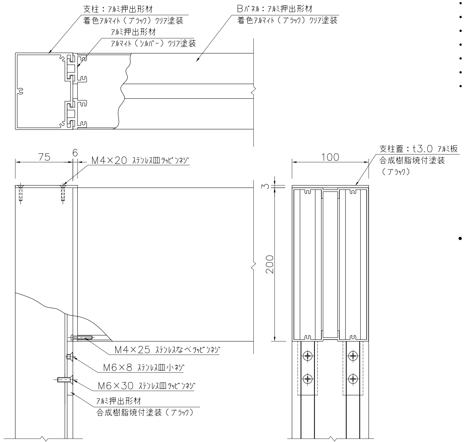
詳細図 S=1/3
