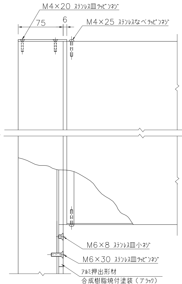
詳細図 S=1/3
