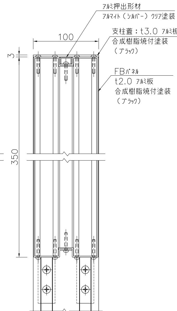
詳細図 S=1/3
