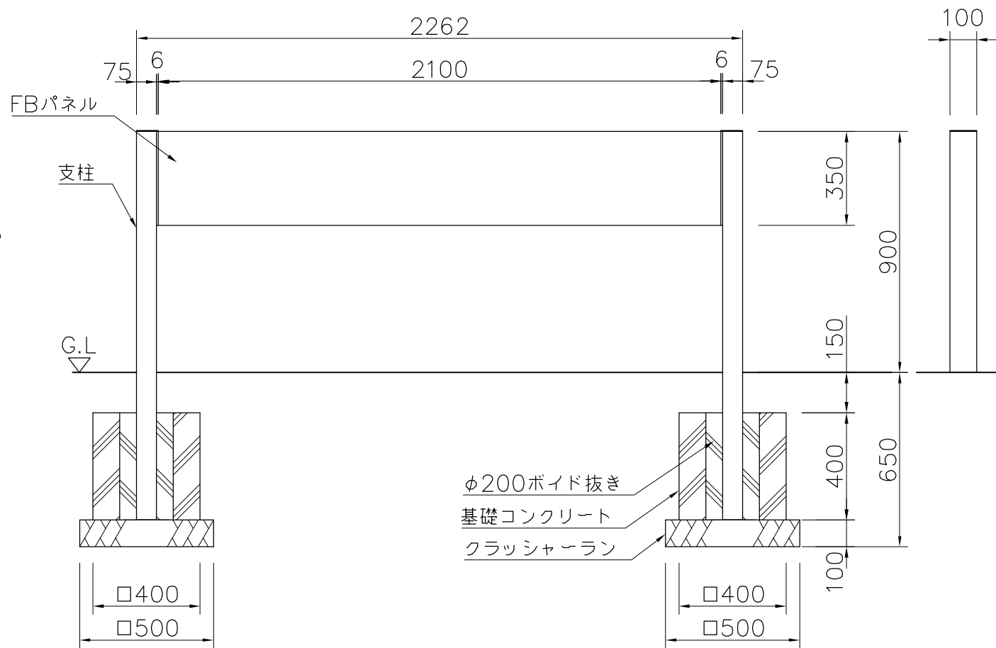
外観図 S=1/20
