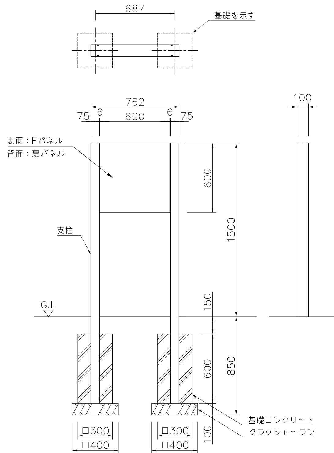
外観図 S=1/20
