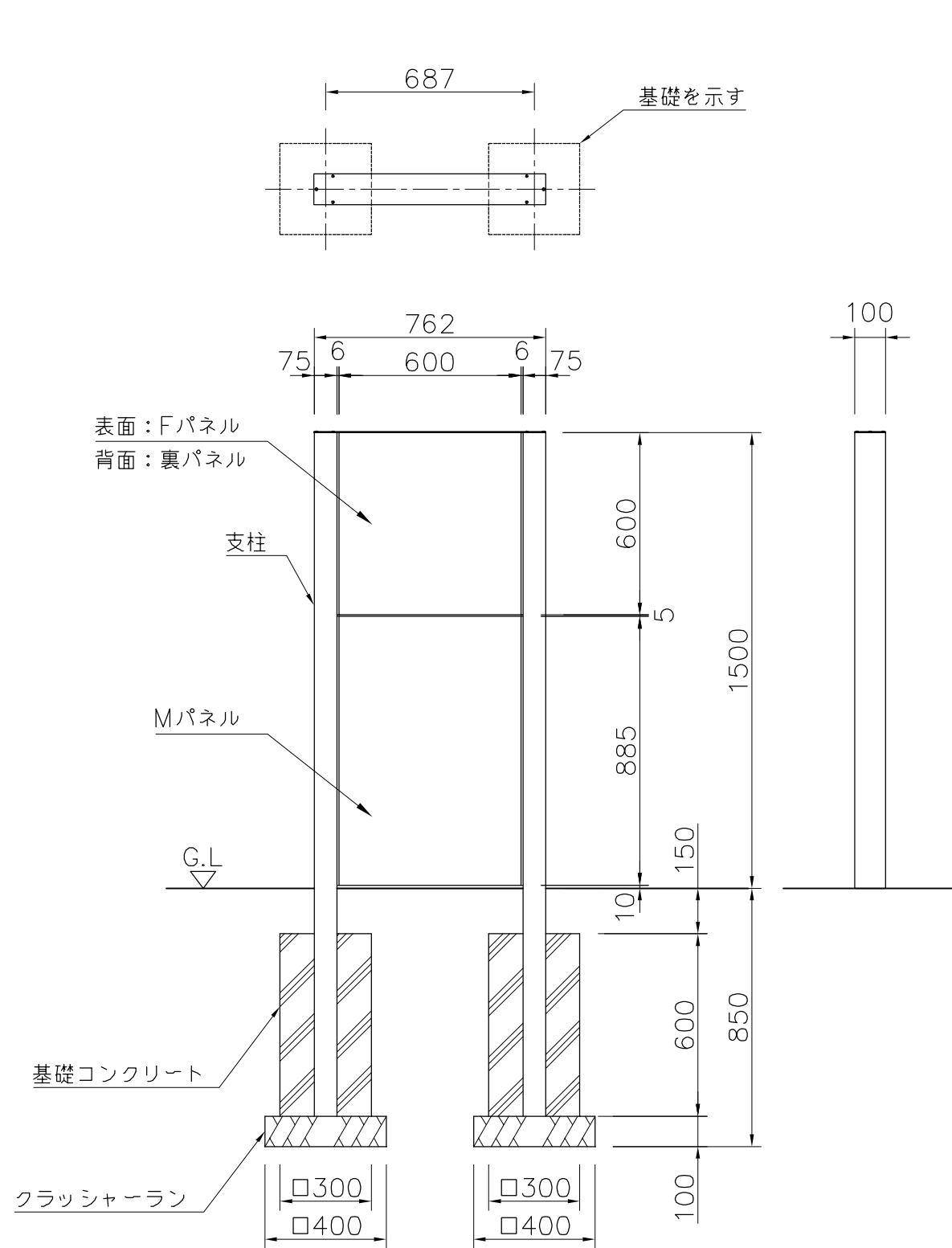
外観図 S=1/20
