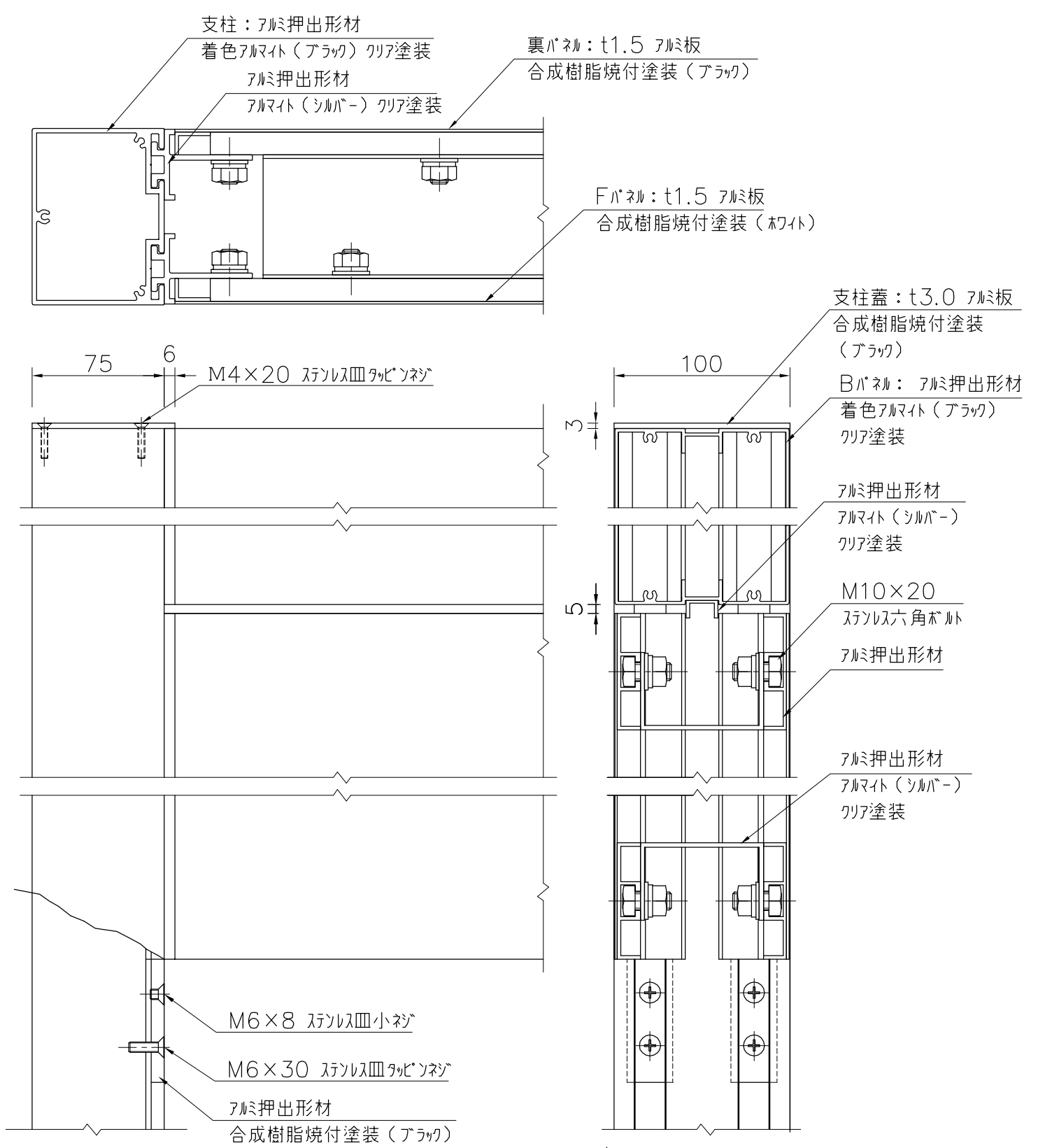
詳細図 S=1/3
