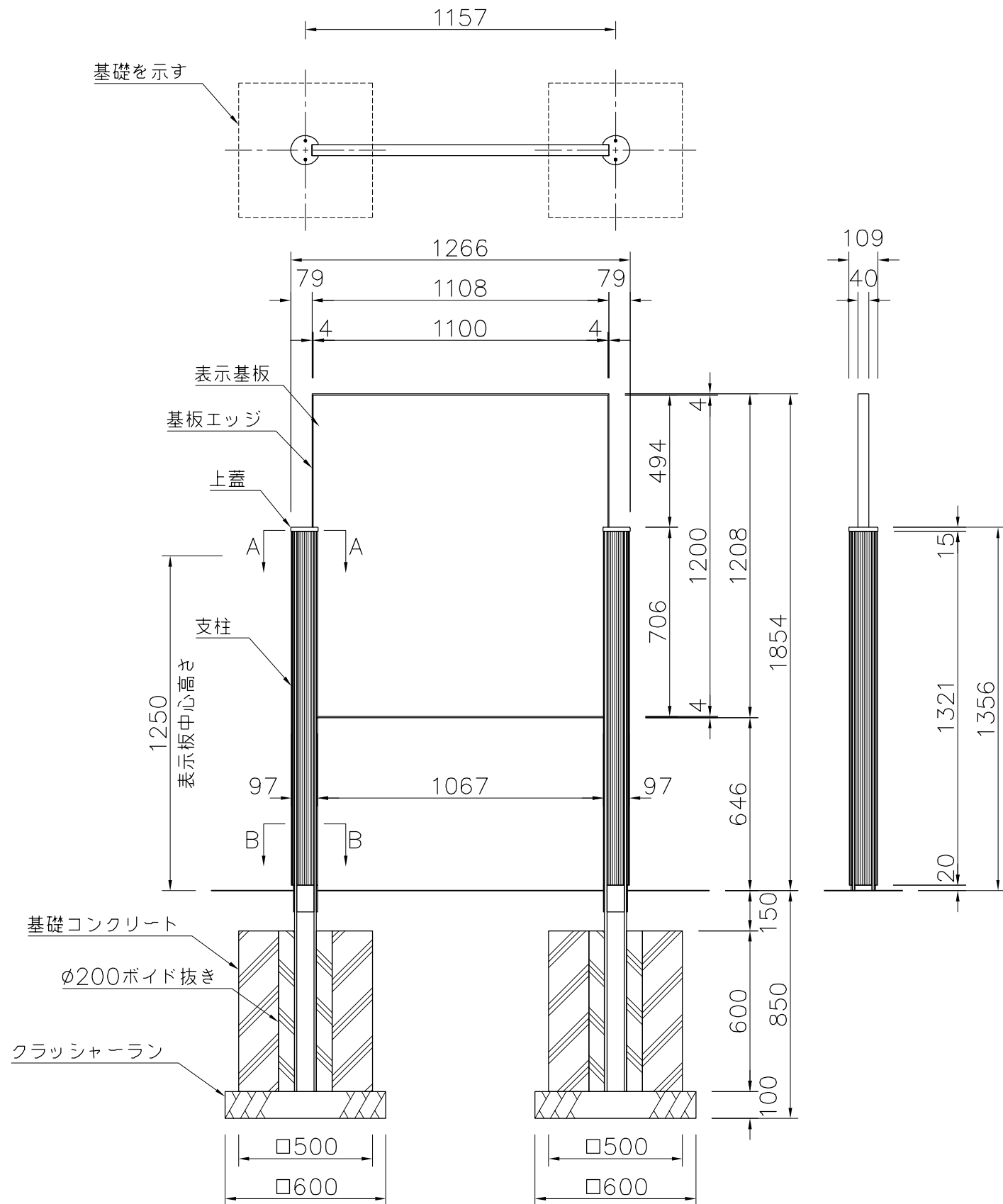
外観図 S=1/20
