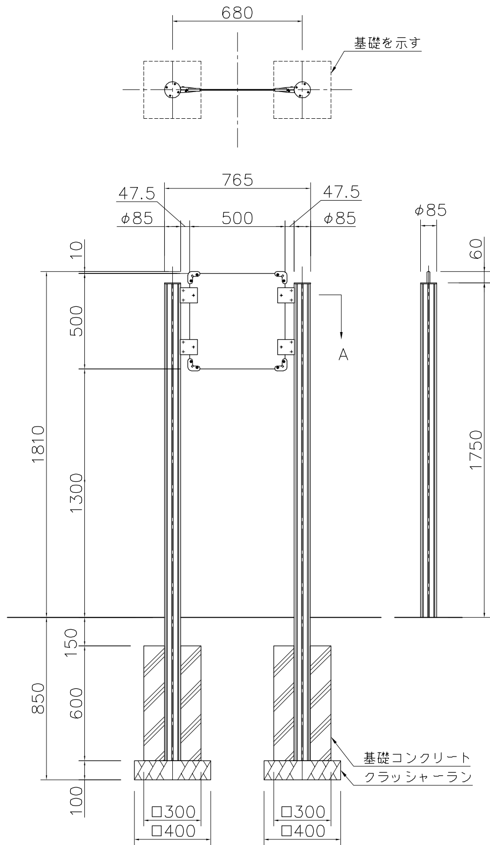
外観図 S=1/20
