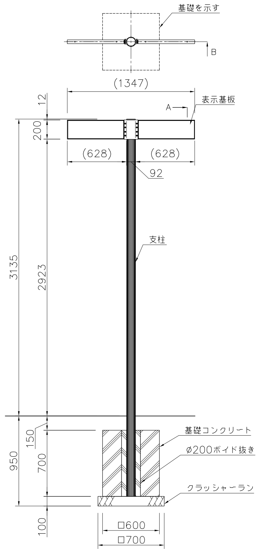
外観図 S=1/25
