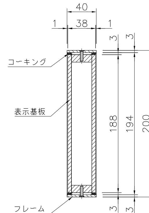
A断面詳細図 S=1/3
