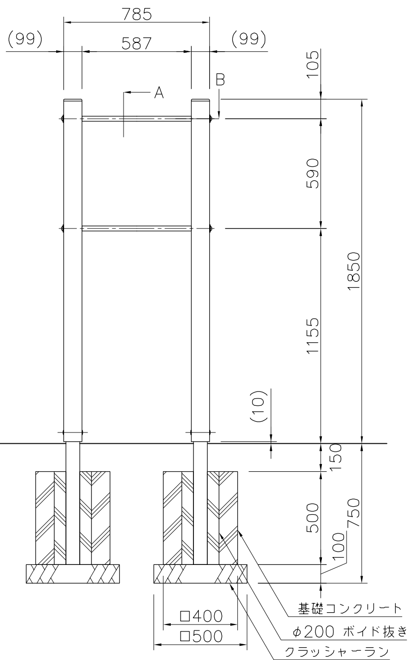
外観図 S=1/20
